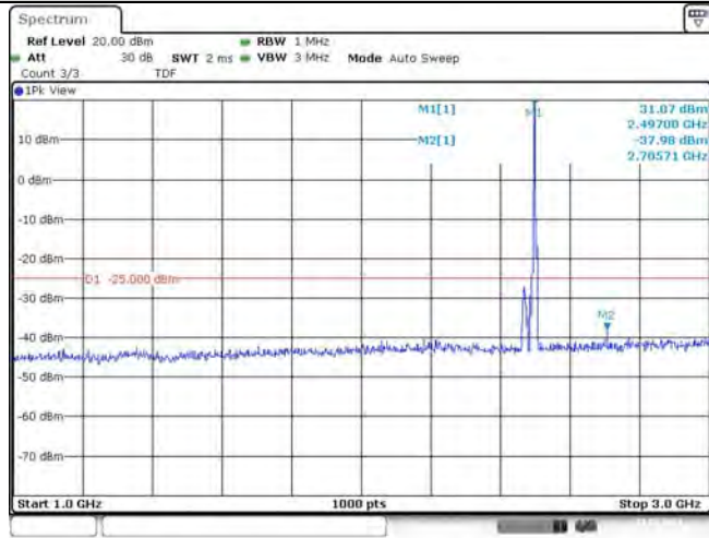
Band41-5MHz-QPSK-39675-1RB#0-Range2:1000~3000MHz
