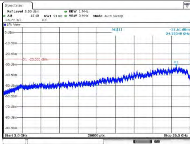
Band41-5MHz-QPSK-39675-1RB#0-Range3:3000~26500MHz
