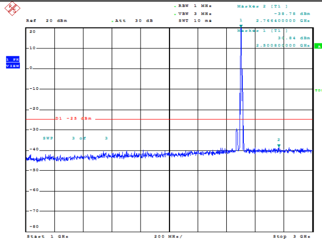
Band7-5MHz-QPSK-20775-1RB#0-Range2:1000~3000MHz
