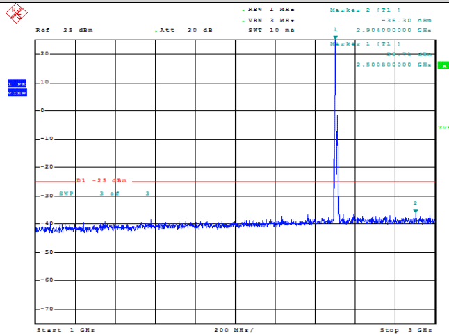
Band7-5MHz-QPSK-20775-1RB#0-Range2:1000~3000MHz
