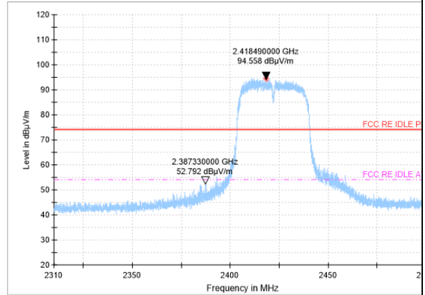
AV detector
