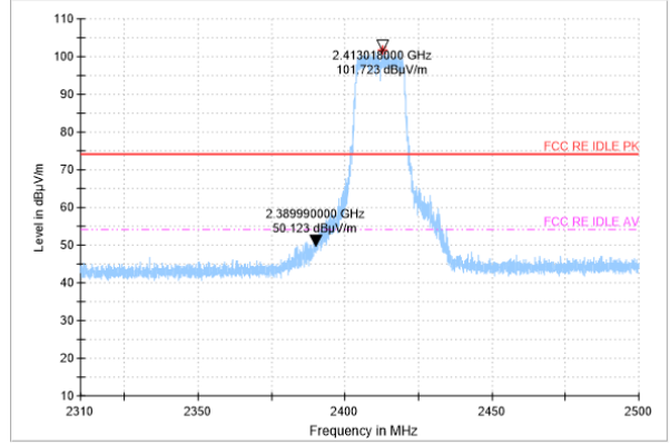
AV detector
