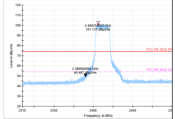
AV detector
