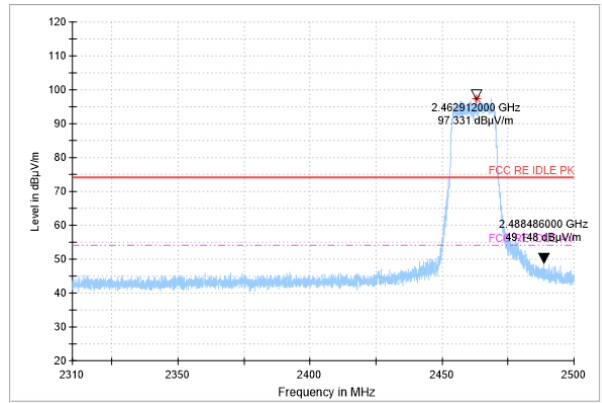
AV detector
