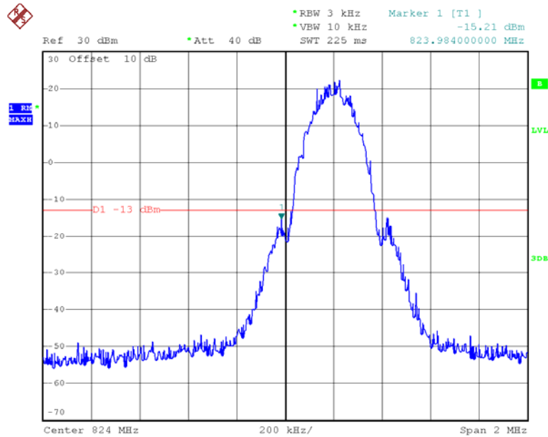
GSM 850, Left Band Edge
