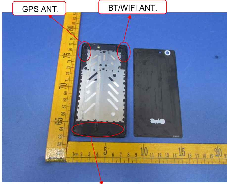
GSM/WCDMA/LTE ANT.
