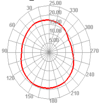
WCDMA_V 4233 TRP H
