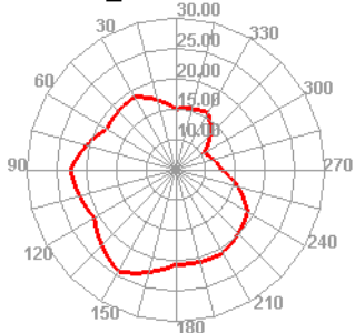
WCDMA_II 9262 TRP E1
