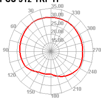
PCS 512 TRP H
