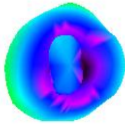
GSM850 128 TRP
