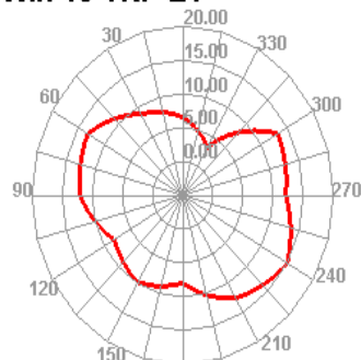
Wifi 13 TRP E1
