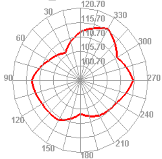
WCDMA_II 9938 TIS E1
