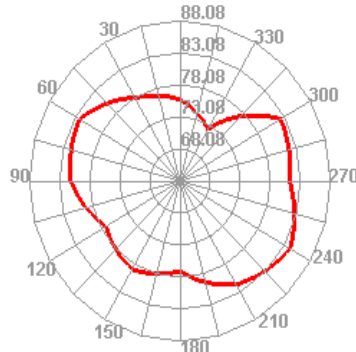
Wifi 13 TIS E1
