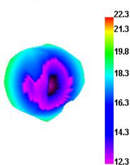
WCDMA_V 4185 TRP
