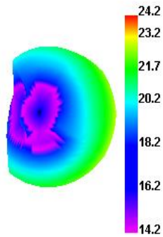
WCDMA_I 9612 TRP
