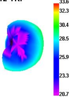
PCS 512 TRP
