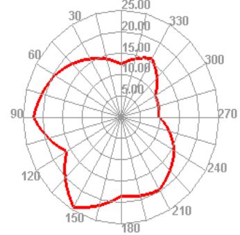
WCDMA_I 9612 TRP E1
