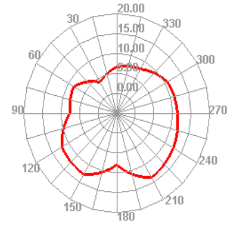
Wifi 13 TRP E2
