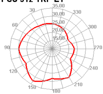
PCS 512 TRP E1
