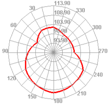
GSM850 251 TIS E2
