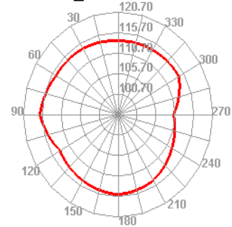
WCDMA_II 9938 TIS H
