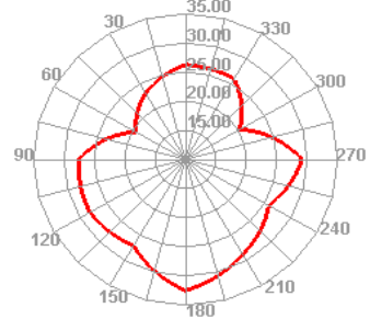
GSM850 251 TRP E1
