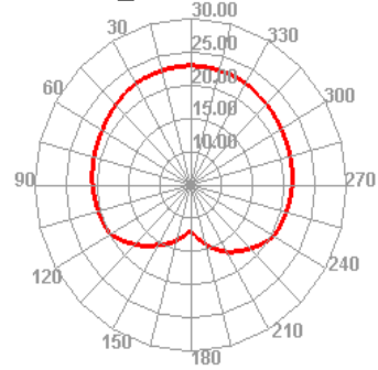
WCDMA_II 9538 TRP H
