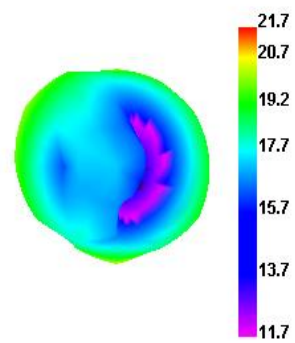
WCDMA_VIII 2863 TRP
