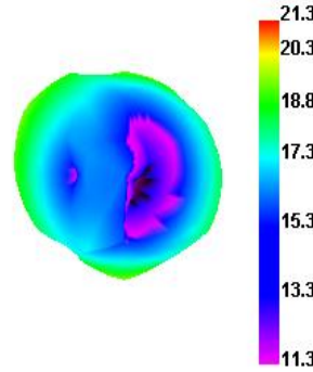
WCDMA_VIII 2788 TRP
