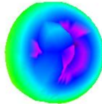
EGSM 1 TRP
