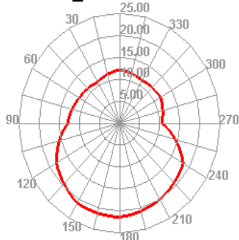
WCDMA_VIII 2788 TRP E2
