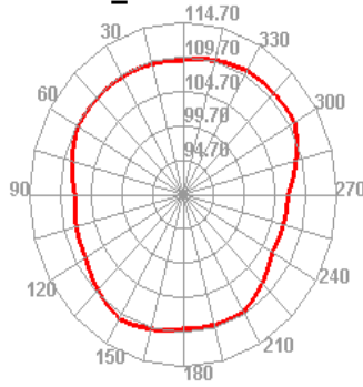
WCDMA_I 10838 TIS H
