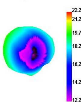
WCDMA_V 4233 TRP
