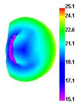
WCDMA_II 9400 TRP
