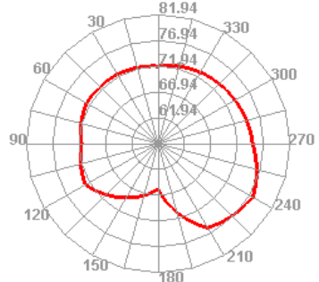
Wifi 165 TIS E2
