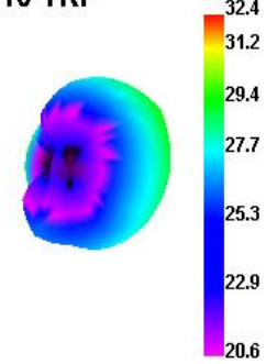
PCS 810 TRP
