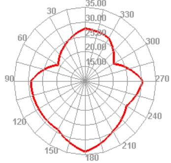
GSM850 190 TRP E1
