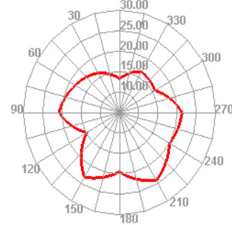
WCDMA_II 9538 TRP E2
