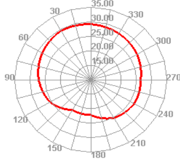
PCS 810 TRP H
