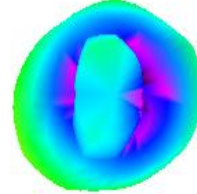
GSM850 251 TRP
