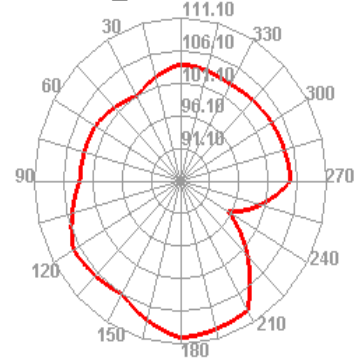
WCDMA_VIII 3088 TIS E1
