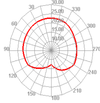
WCDMA_II 9262 TRP H
