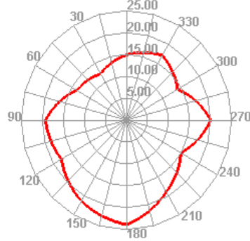
WCDMA_V 4132 TRP E1
