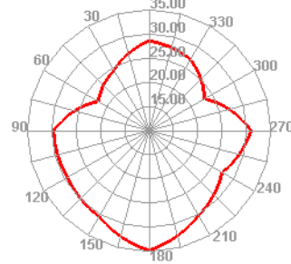
GSM850 128 TRP E1
