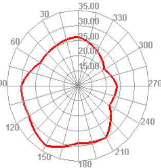
DCS 885 TRP E1
