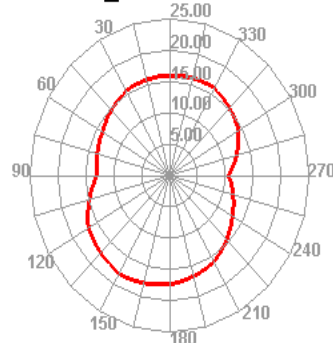
WCDMA_VIII 2863 TRP H
