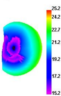
WCDMA_II 9538 TRP
