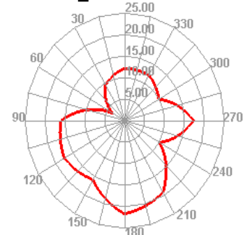
WCDMA_VIII 2863 TRP E1
