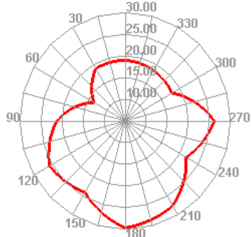
EGSM 62 TRP E1
