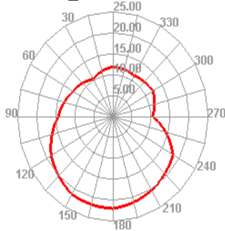
WCDMA_VIII 2712 TRP E2
