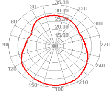
GSM850 190 TRP E2
