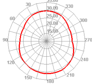
GSM850 128 TRP H
