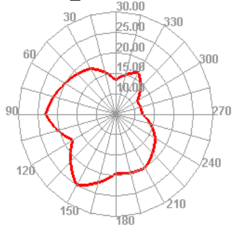
WCDMA_II 9538 TRP E1
