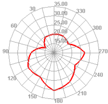
EGSM 1 TRP E1
