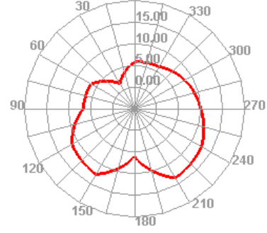
Wifi 6 TRP E2
