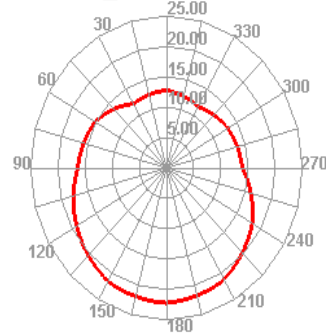
WCDMA_V 4233 TRP E2
