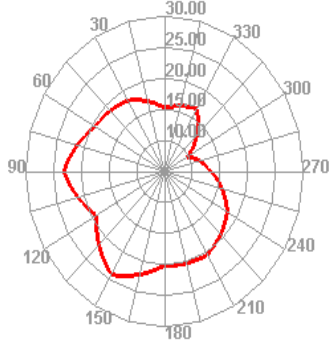
WCDMA_II 9400 TRP E1
