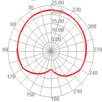
WCDMA_I 9612 TRP H
