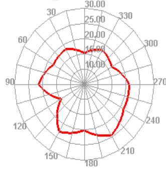
WCDMA_II 9400 TRP E2
