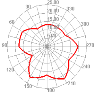
WCDMA_I 9750 TRP E2
