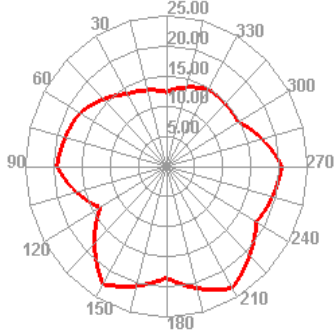
WCDMA_I 9612 TRP E2
