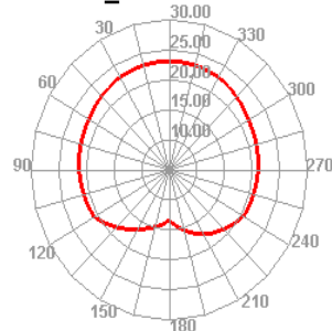
WCDMA_II 9400 TRP H
