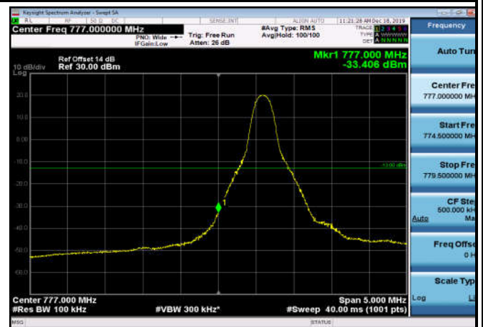
LowRange_FDD13_10MHz_782_OneRB_low_QPSK
