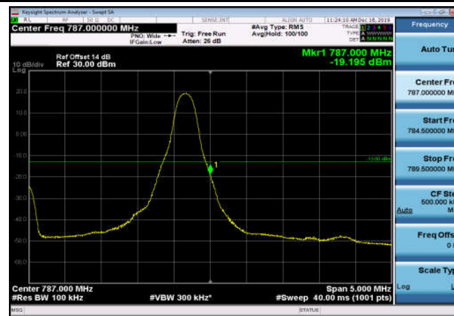
HighRange_FDD13_5MHz_784.5_OneRB_high_Q16
