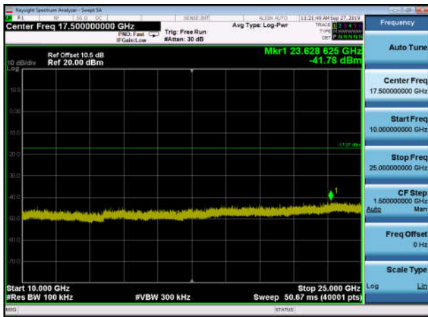
,Plot 5,10000MHz~25000MHz-802.11n(HT20),2462MHz
