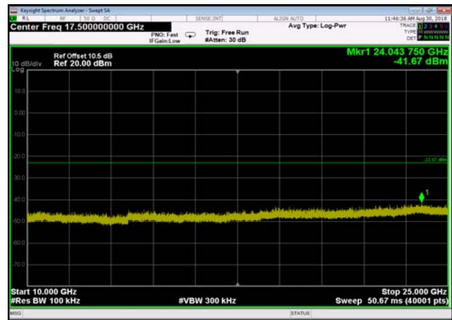
,Plot 5,10000MHz~25000MHz-802.11n(HT40),2452MHz
