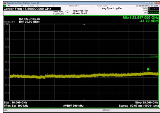
,Plot 5,10000MHz~25000MHz-802.11n(HT40),2452MHz
