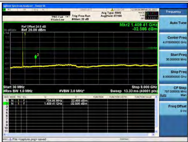
Band17 / 10MHz / Low CH / 16QAM
