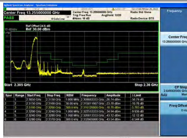
Band40 / 10MHz / High CH / QPSK / 1 RB
