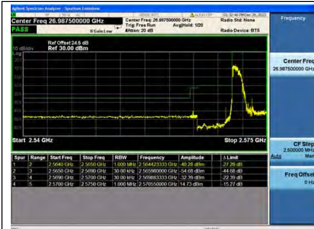
Band38 / 5MHz / Low CH / QPSK / 1 RB
