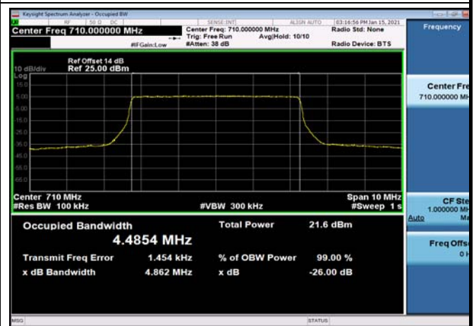
FDD17_MidRange_5_710_Q16
