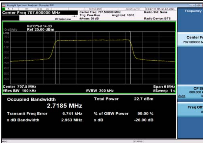
FDD12_MidRange_3MHz_707.5MHz_QPSK
