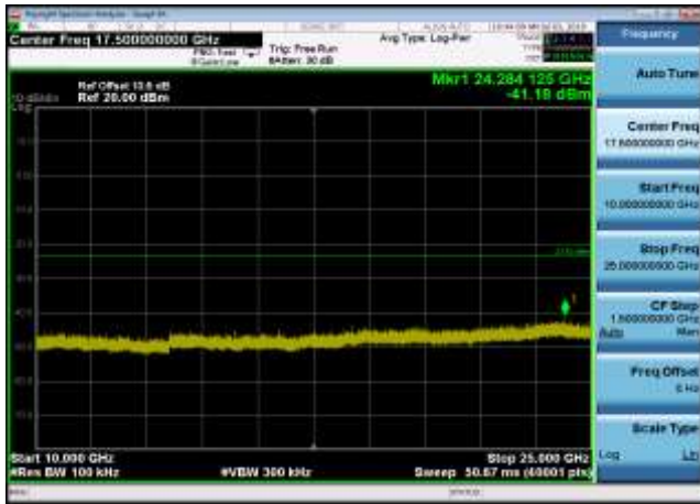
,Plot 5,10000MHz~25000MHz-802.11n(HT20),2462MHz
