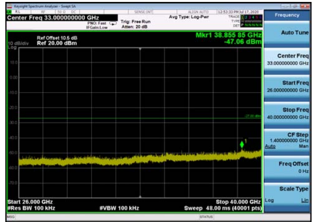
U-NII-3 ,Plot 2,26000MHz~40000MHz-802.11n(40MHz),5795MHz,Ant1
