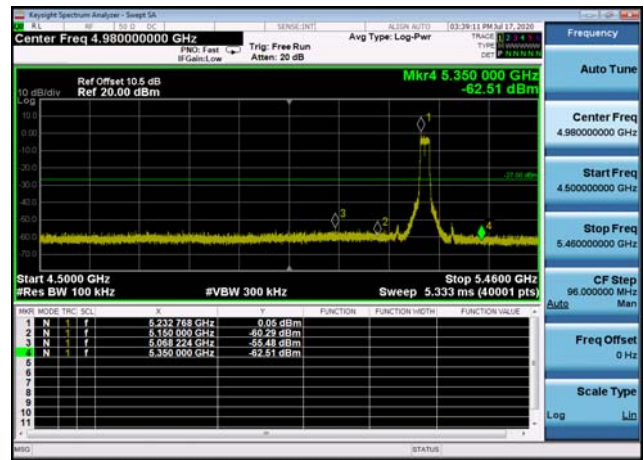
U-NII-1 Band Edge-802.11ac(40MHz) ,5230MHz,Ant1
