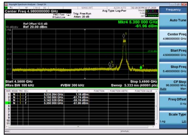
U-NII-1 Band Edge-802.11n(40MHz) ,5230MHz,Ant1
