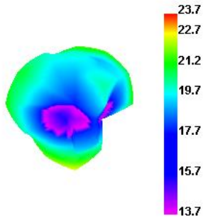
WCDMA_II 9400 TRP
