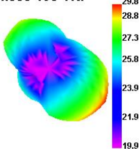
GSM850 190 TRP
