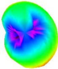
EGSM 62 TRP
