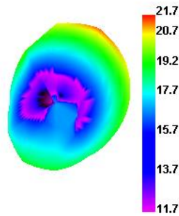
WCDMA_VIII 2788 TRP
