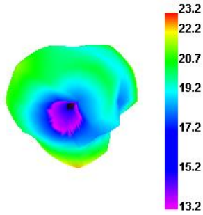
WCDMA_I 9750 TRP
