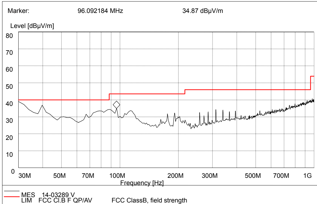
(Plot A: 30MHz to 1GHz, Antenna Vertical)
