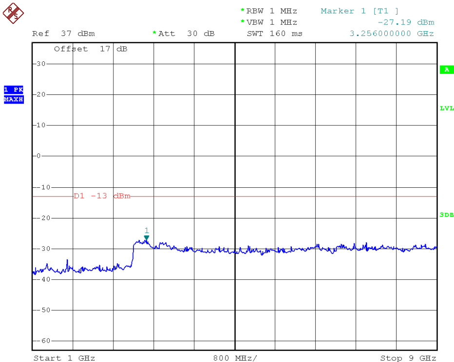
1GHz~9GHz
