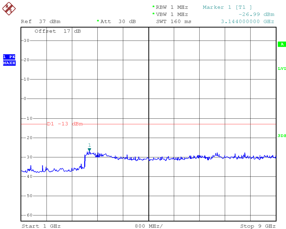
1GHz~9GHz
