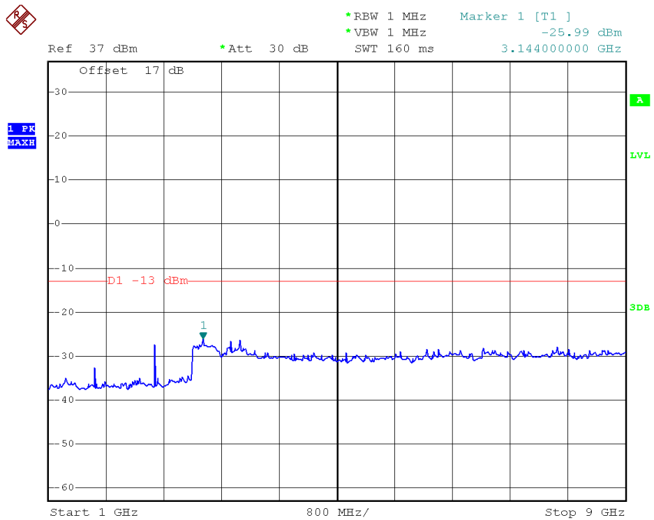
1GHz~9GHz
