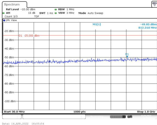
Band38-20MHz-16QAM-37850-100RB#0-Range2:1000~3000MHz
