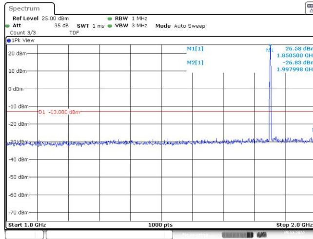
Band25-1.4MHz-QPSK-26047-1RB#0-Range2:1000~2000MHz
