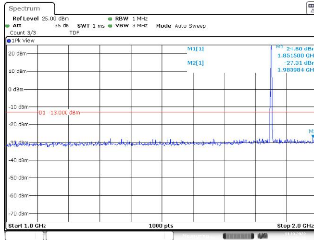
Band2-1.4MHz-QPSK-18607-6RB#0-Range2:1000~2000MHz
