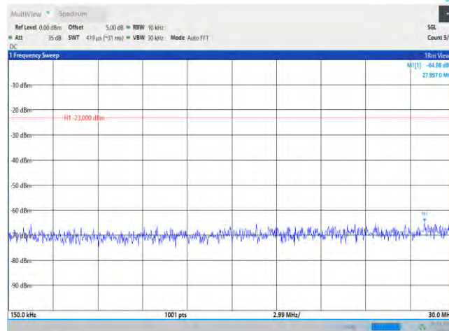
Band66-20MHz-QPSK-132072-1RB#0-Range2:0.15~30MHz
