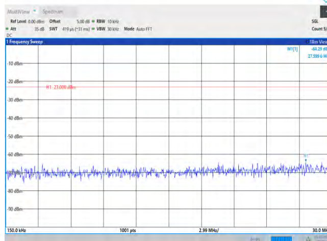
Band26-10MHz-QPSK-26740-1RB#0-Range2:0.15~30MHz
