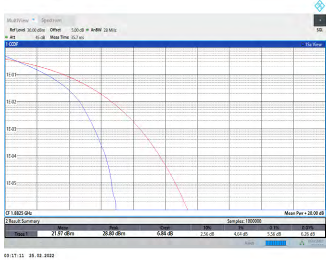
Band25-20MHz-QPSK-26365-100RB#0
