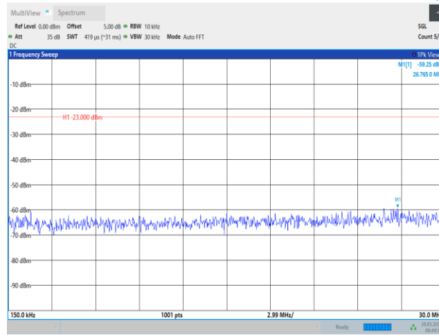
Band13-10MHz-QPSK-23230-1RB#0-Range2:0.15~30MHz
