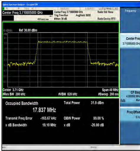
1-N78-3700-3800-30-20-L-1-DFT-QPSK-Outer_Full-50@0-Ant1-17.837-19.10-≤20-PASS
