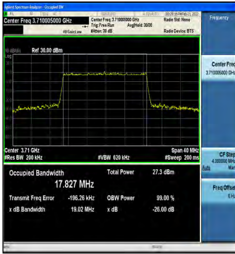
1-N77-3700-3980-30-20-L-5-DFT-256QAM-Outer_Fu II-50@0-Ant1-17.827-19.02-≤20-PASS
