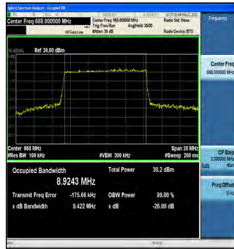
1-N71-15-10-L-3-DFT-16QAM-Outer_Full-50@0-Ant 1-8.9243-9.422-≤10-PASS
