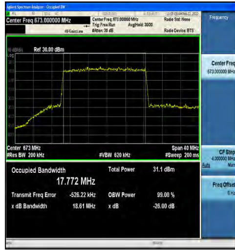
1-N71-15-20-L-1-DFT-QPSK-Outer_Full-100@0-Ant 1-17.772-18.61-≤20-PASS
