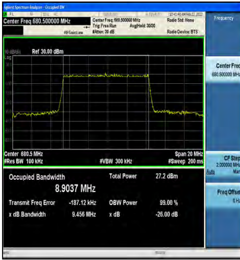
1-N71-15-10-M-5-DFT-256QAM-Outer_Full-50@0-A nt1-8.9037-9.456-≤10-PASS
