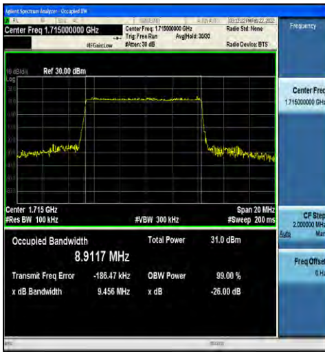
1-N66-15-10-L-2-DFT-PI2BPSK-Outer_Full-50@0-A nt1-8.9117-9.456-≤10-PASS
