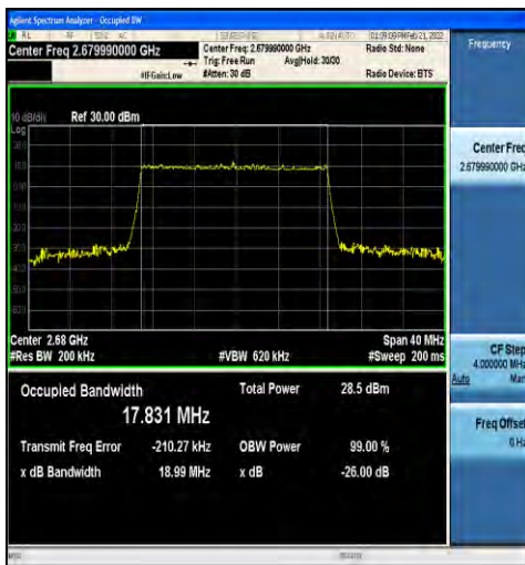
1-N41-30-20-H-5-DFT-256QAM-Outer_Full-50@0-A nt1-17.831-18.99-≤20-PASS
