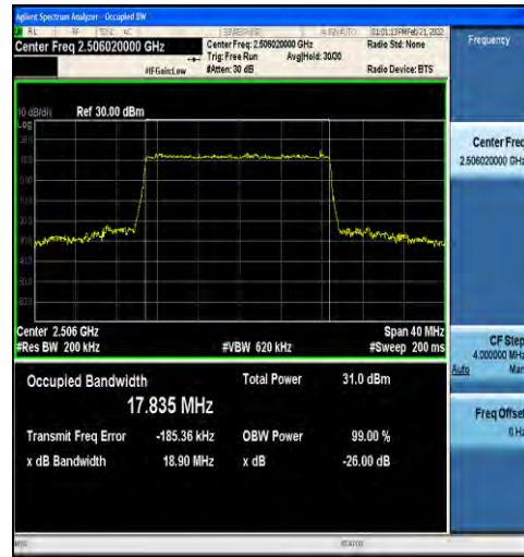
1-N41-30-20-L-2-DFT-PI2BPSK-Outer_Full-50@0-A nt1-17.835-18.90-≤20-PASS
