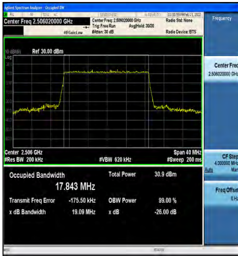
1-N41-30-20-L-1-DFT-QPSK-Outer_Full-50@0-Ant1- 17.843-19.09-≤20-PASS
