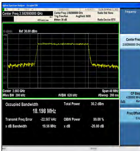
1-N41-30-20-M-6-CP-QPSK-Outer_Full-51@0-Ant1 18.198-19.56-≤20-PASS
