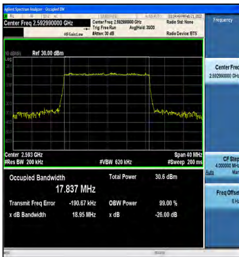
1-N41-30-20-M-2-DFT-P12BPSK-Outer_Full-50@0-A nt1-17.837-18.95-≤20-PASS
