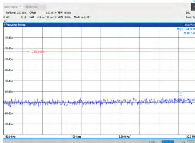
Band2-20MHz-QPSK-18700-1RB#0-Range2:0.15~30MHz
