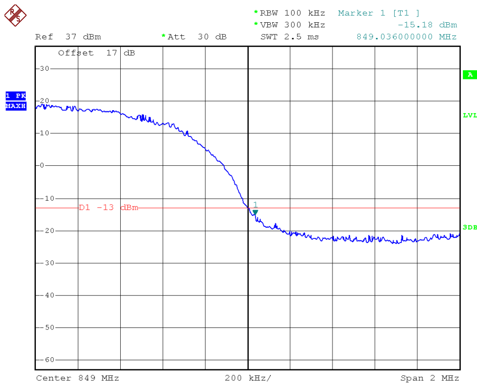
(Plot J: WCDMA 850 Channel = 4233)
