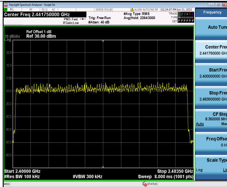
\pi/4 DQPSK Modulation
