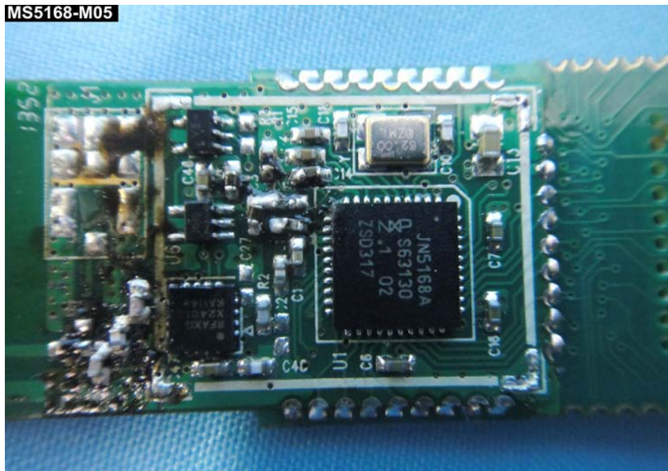
EUT Photo 5 )
