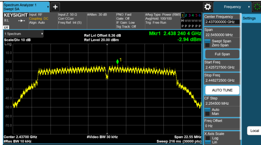
11G-SISO_Ant2_2437
