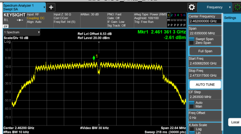
11G-SISO_Ant2_2462
