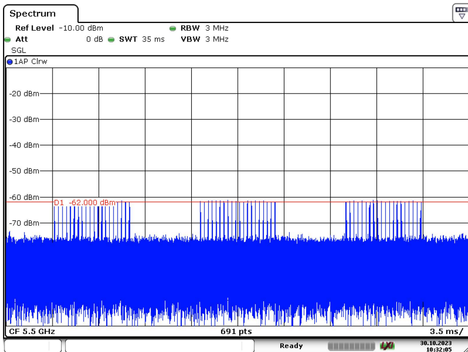
Radar Type 4 – 5500MHz
