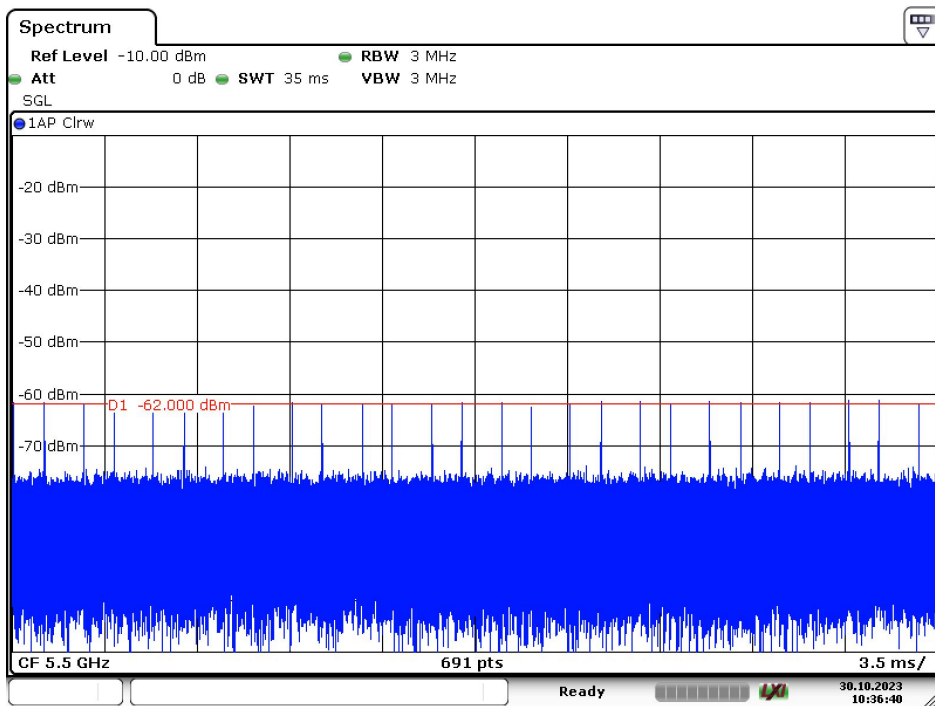
Radar Type 6 – 5500MHz
