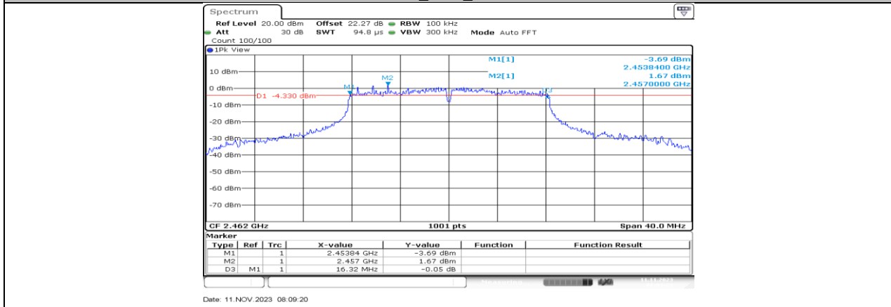
11G_Ant1_2462
