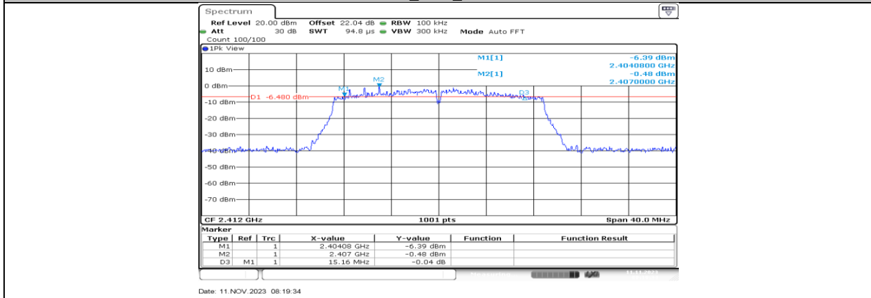
11N20MIMO_Ant0_2412
