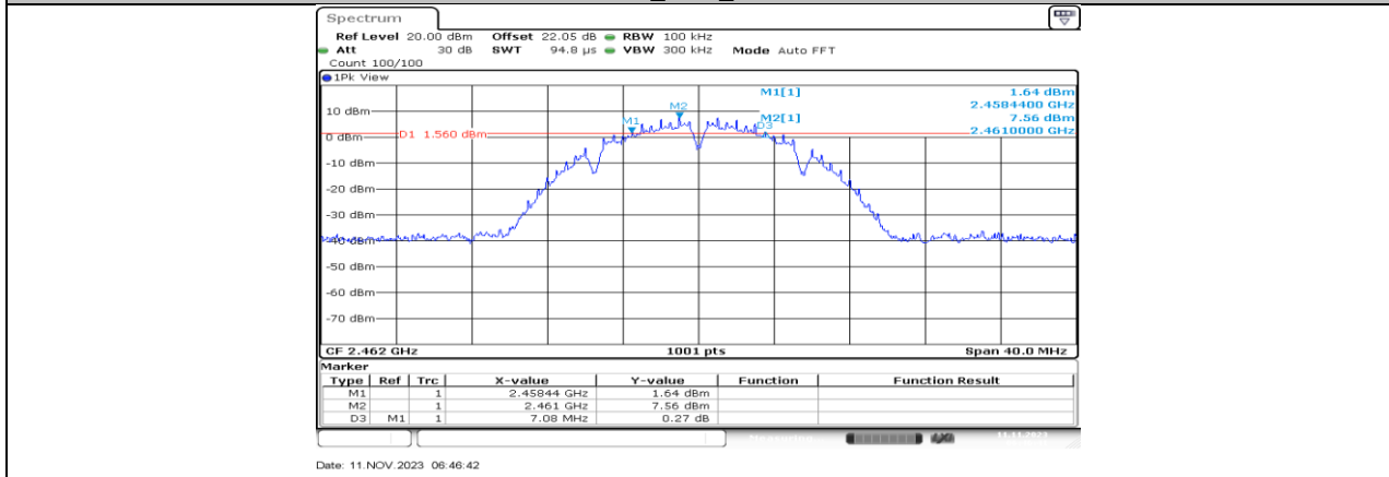
11B_Ant0_2462
