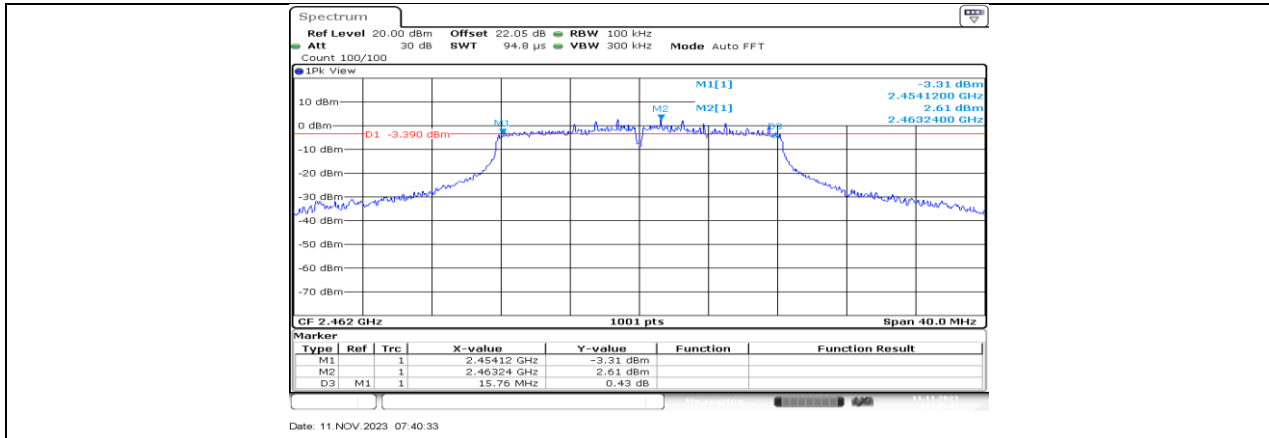
11G_Ant0_2462
