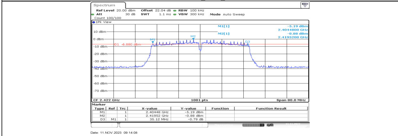
11N40MIMO_Ant0_2422
