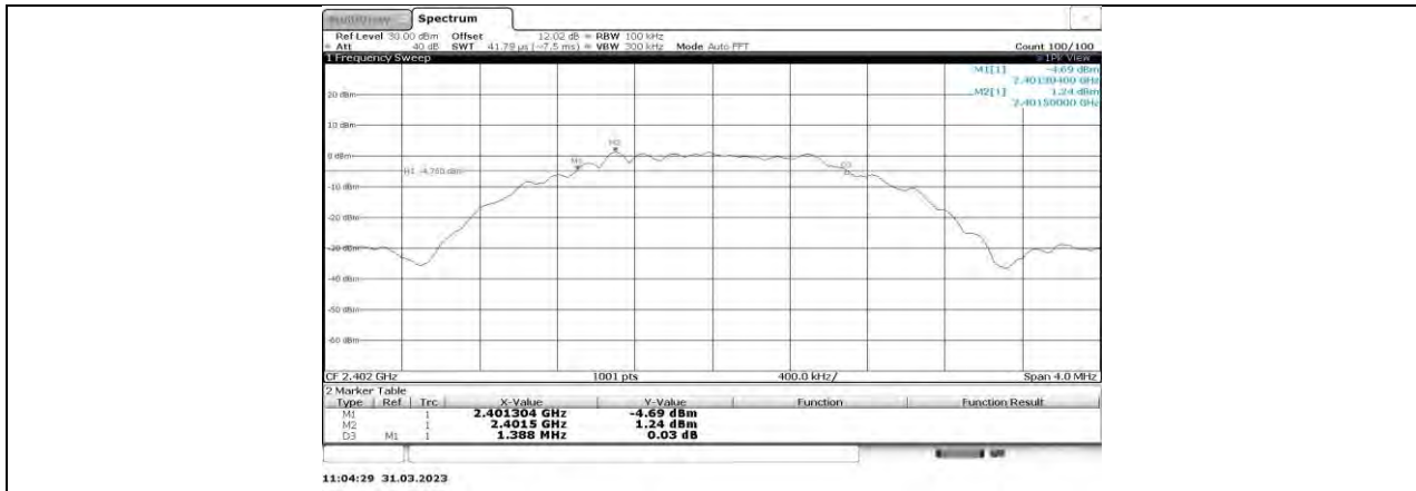
BLE 2M Ant1 2402
