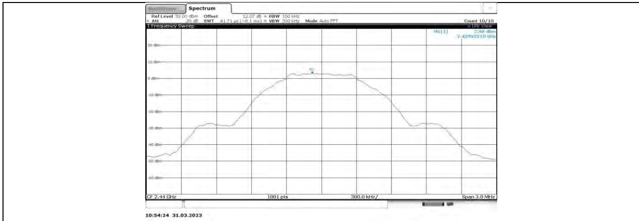
BLE 1M Ant1 2440 0~Reference
