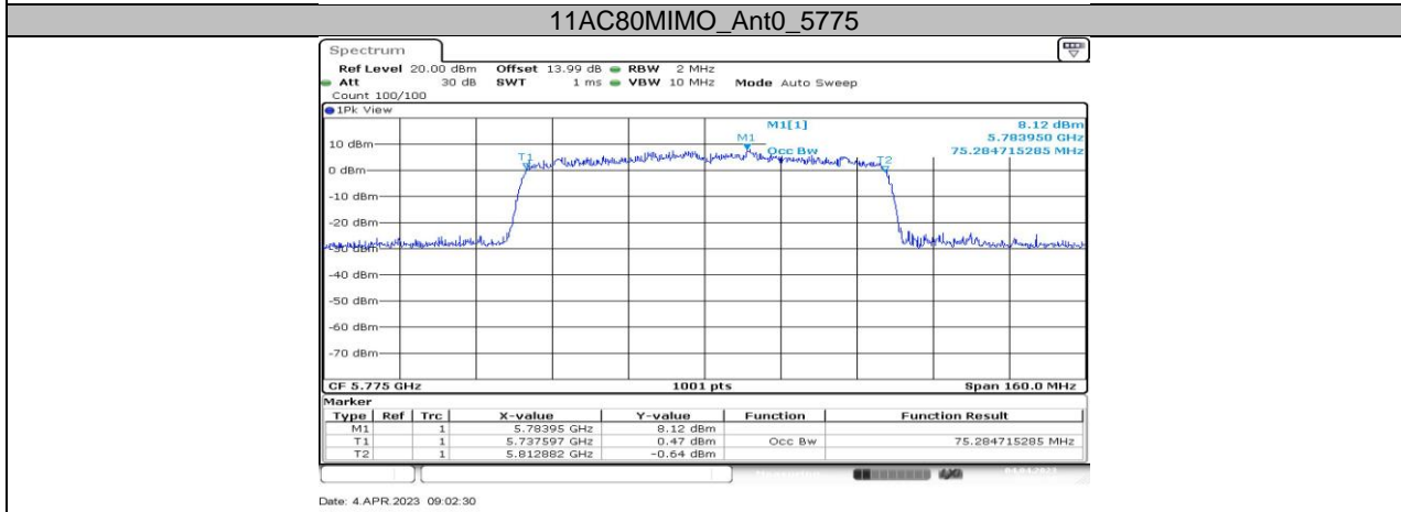
11AC80MIMO_Ant1_5775
