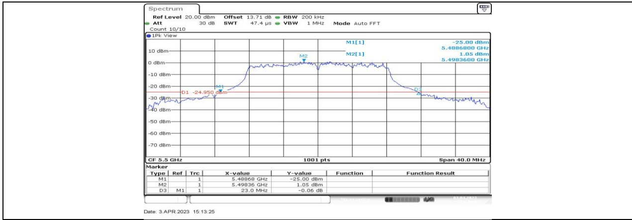
11A_Ant0_5500
