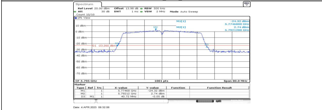
11N40MIMO_Ant0_5795
