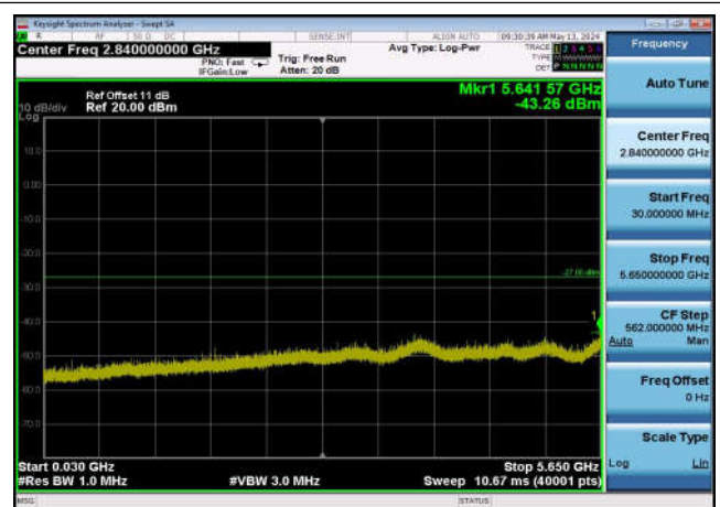
U-NII-3 ,Plot 2,30MHz~5650MHz-802.11n (40MHz),5755MHz,Ant0
