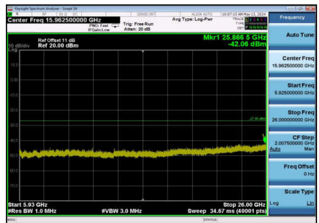
U-NII-3 ,Plot 3,5925MHz~26000MHz-802. 11ax(80MHz),5775MHz,Ant0
