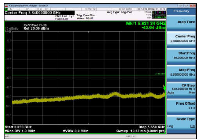
U-NII-3 ,Plot 2,30MHz~5650MHz-802.11a x(20MHz),5745MHz,Ant0
