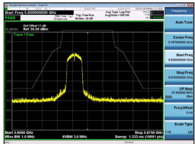
U-NII-3 ,Plot 1,Band Edge-802.11ac(80 MHz),5775MHz,Ant0
