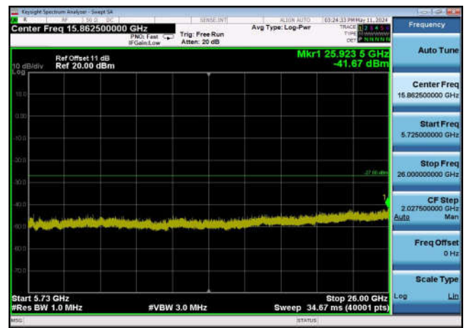
U-NII-2c ,Plot 3,5725MHz~26000MHz-802 .11ac(20MHz),5700MHz,Ant0
