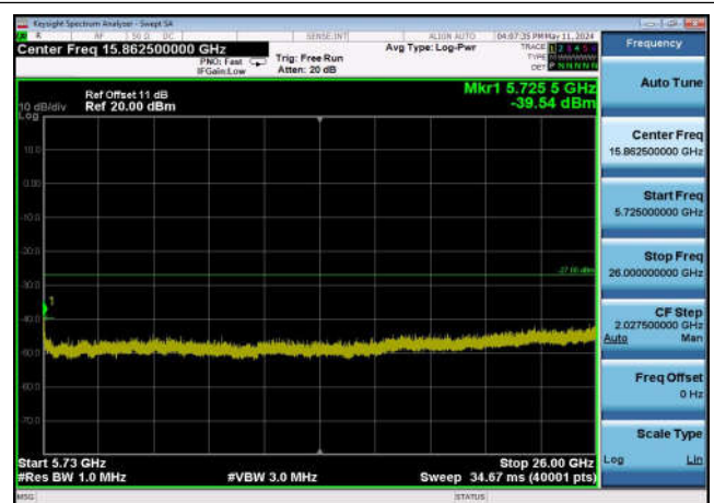
U-NII-2c ,Plot 3,5725MHz~26000MHz-802 .11ax(20MHz),5700MHz,Ant0
