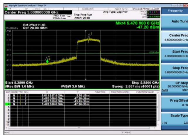
U-NII-2c ,Plot 1,Band Edge-802.11ax(2 0MHz),5600MHz,Ant0
