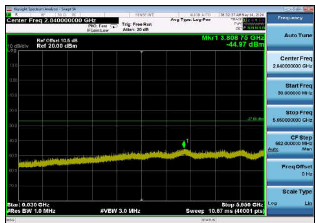
U-NII-3 ,Plot 2,30MHz~5650MHz-802.11n (20MHz),5825MHz,Ant0
