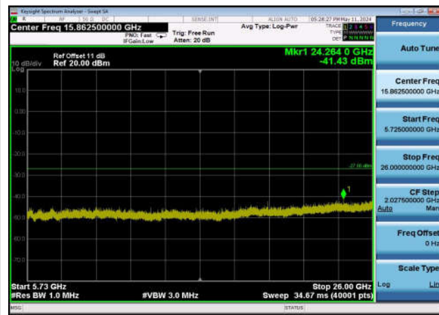
U-NII-2c ,Plot 3,5725MHz~26000MHz-802 .11ax(40MHz),5670MHz,Ant0
