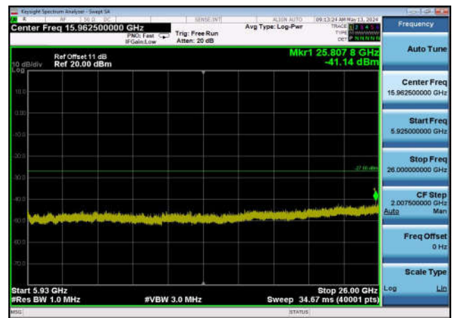
U-NII-3 ,Plot 3,5925MHz~26000MHz-802. 11ax(40MHz),5755MHz,Ant0
