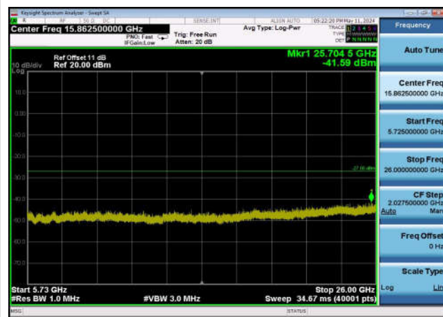
U-NII-2c ,Plot 3,5725MHz~26000MHz-802 .11ac(80MHz),5610MHz,Ant0
