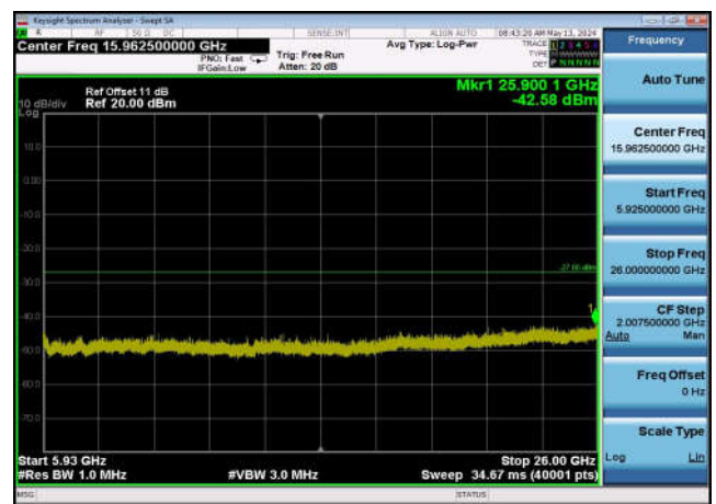
U-NII-3 ,Plot 3,5925MHz~26000MHz-802. 11ac(40MHz),5755MHz,Ant0
