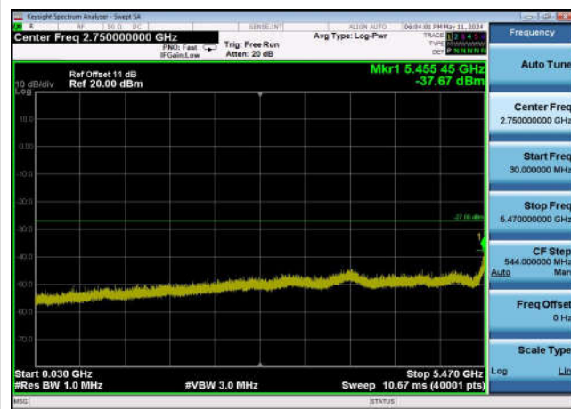
U-NII-2c ,Plot 2,30MHz~5470MHz-802.11 ax(20MHz),5500MHz,Ant0
