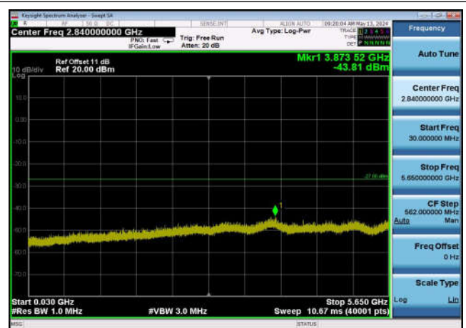
U-NII-3 ,Plot 2,30MHz~5650MHz-802.11a x(20MHz),5825MHz,Ant0
