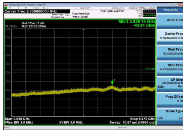
U-NII-2c ,Plot 2,30MHz~5470MHz-802.11 ax(80MHz),5530MHz,Ant0
