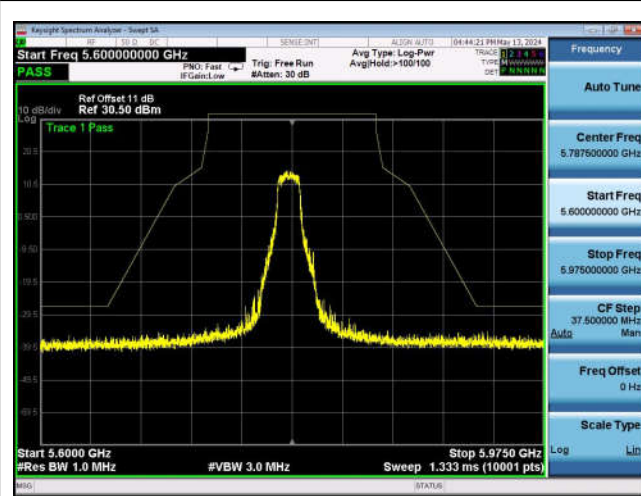
U-NII-3 ,Plot 1,Band Edge-802.11a(20MHz),5785MHz,Ant0
