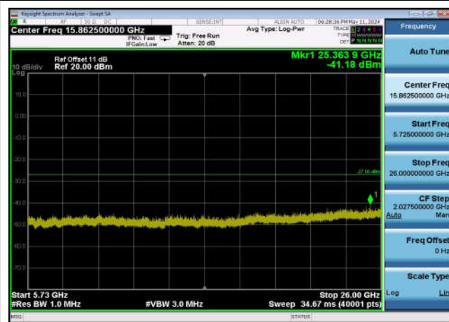
U-NII-2c ,Plot 3,5725MHz~26000MHz-802 .11ax(80MHz),5610MHz,Ant0
