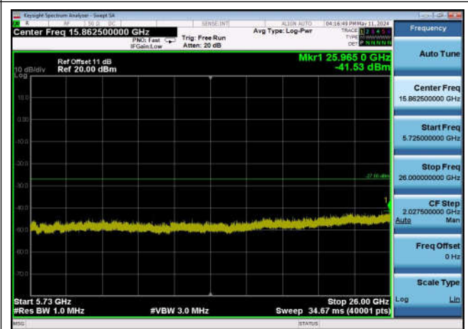
U-NII-2c ,Plot 3,5725MHz~26000MHz-802.11n(40MHz),5510MHz,Ant0
