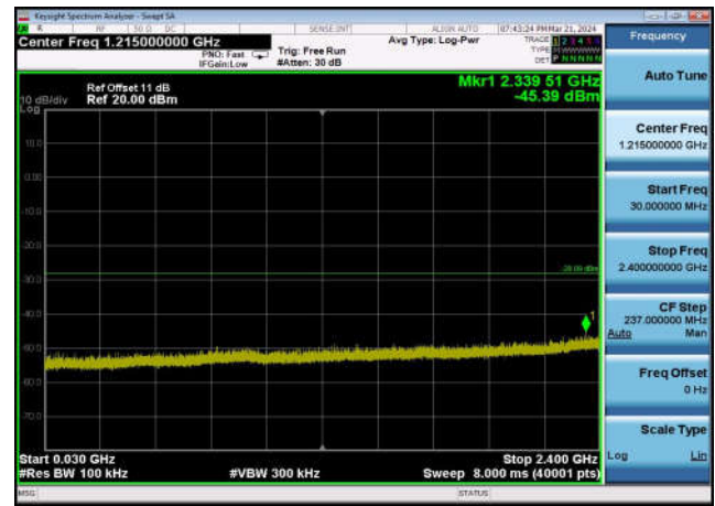
,Plot 3,30MHz~2400MHz-802.11n(20MHz),2462MHz,Ant1
