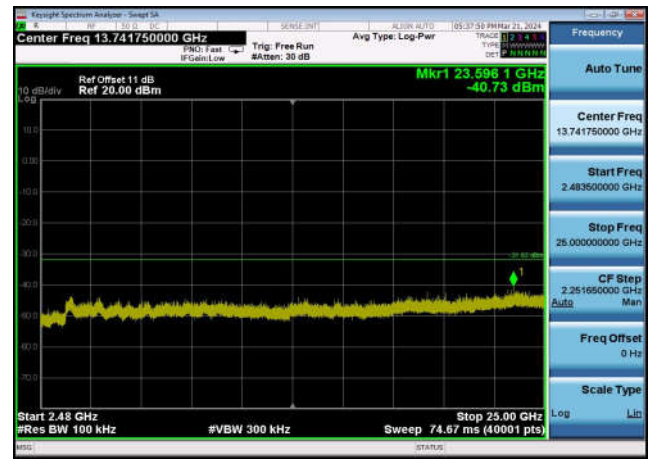
,Plot 4,2483.5MHz~25000MHz-802.11ax(4 0MHz),2452MHz,Ant1
