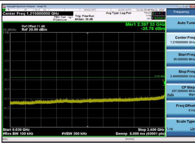
,Plot 3,30MHz~2400MHz-802.11n(20MHz),2437MHz,Ant0
