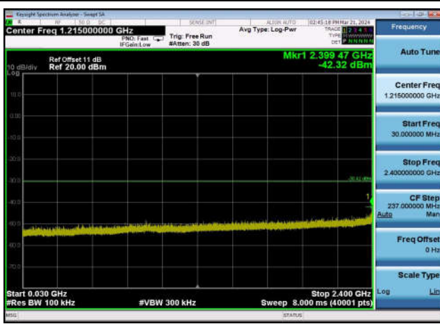
,Plot 3,30MHz~2400MHz-802.11ax(40MHz) ,2437MHz,Ant0
