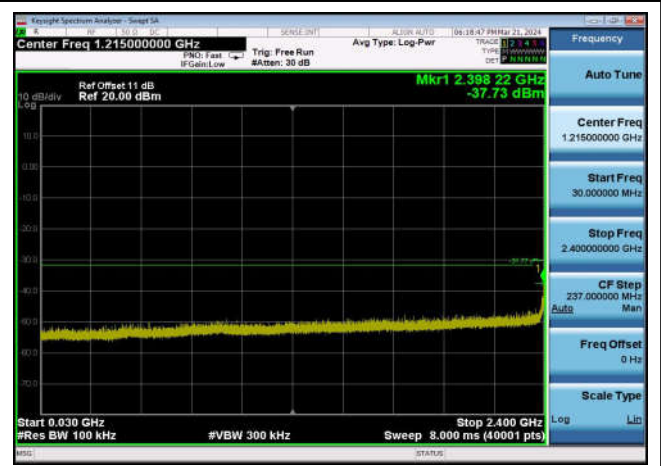
,Plot 3,30MHz~2400MHz-802.11ax(40MHz) ,2437MHz,Ant1
