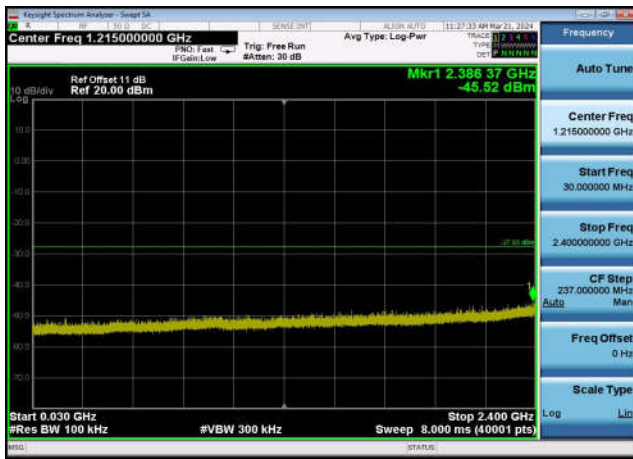
,Plot 3,30MHz~2400MHz-802.11n(20MHz),2462MHz,Ant0
