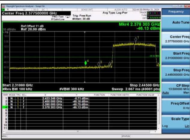
,Plot 2,Band Edge-802.11ax(40MHz) ,2437MHz,Ant0
