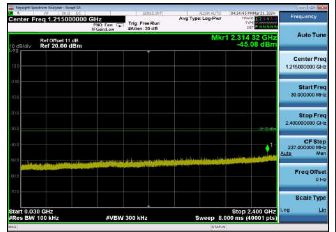
,Plot 3,30MHz~2400MHz-802.11n(40MHz),2452MHz,Ant1
