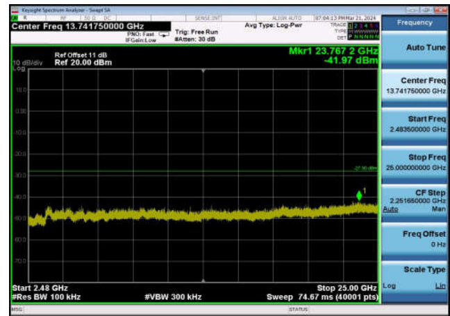
,Plot 4,2483.5MHz~25000MHz-802.11ax(4 0MHz),2422MHz,Ant1
