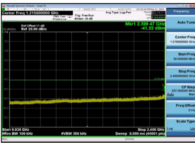
,Plot 3,30MHz~2400MHz-802.11n(40MHz),2437MHz,Ant0
