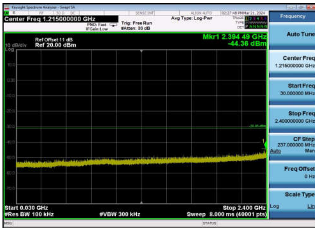
,Plot 3,30MHz~2400MHz-802.11ax(40MHz) ,2452MHz,Ant0
