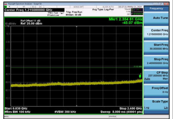
,Plot 3,30MHz~2400MHz-802.11ax(40MHz) ,2452MHz,Ant1
