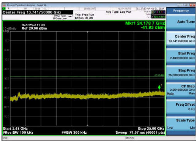
,Plot 4,2483.5MHz~25000MHz-802.11n(20 MHz),2462MHz,Ant0
