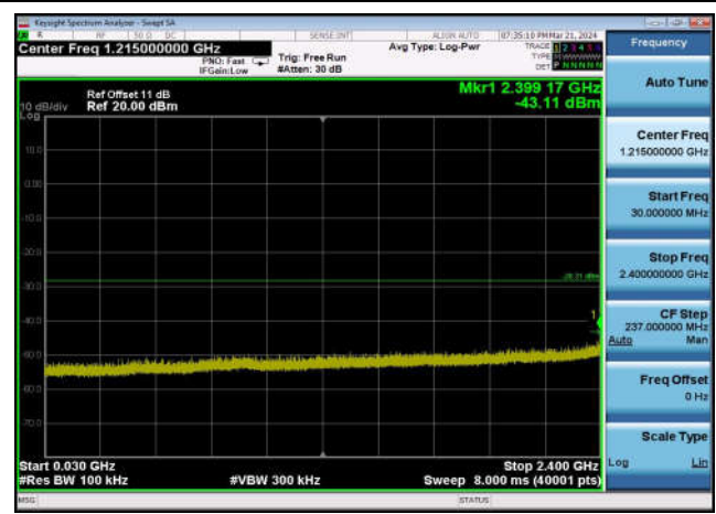
,Plot 3,30MHz~2400MHz-802.11n(20MHz),2437MHz,Ant1
