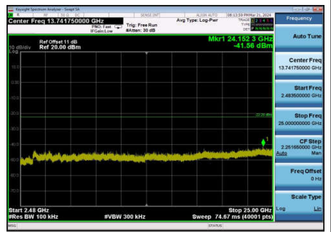
,Plot 4,2483.5MHz~25000MHz-802.11b ,2437MHz,Ant1
