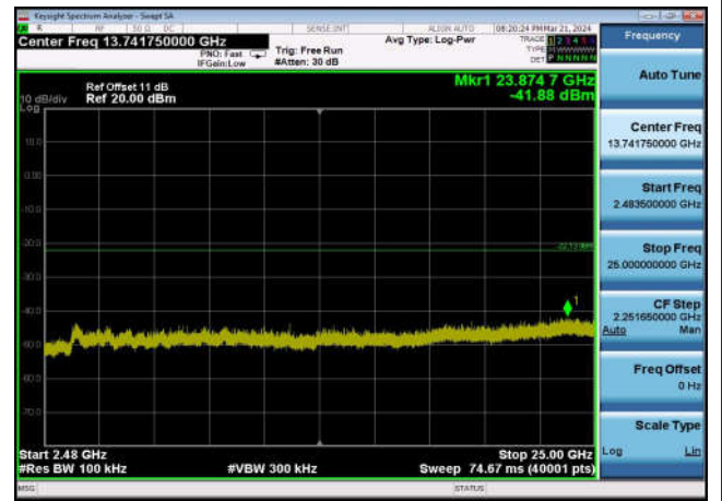
,Plot 4,2483.5MHz~25000MHz-802.11b ,2462MHz,Ant1
