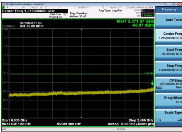
,Plot 3,30MHz~2400MHz-802.11n(40MHz),2452MHz,Ant0
