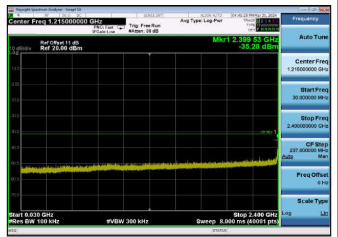
,Plot 3,30MHz~2400MHz-802.11n(40MHz),2437MHz,Ant1
