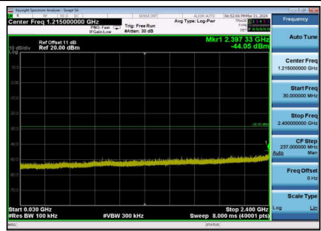
,Plot 3,30MHz~2400MHz-802.11ax(20MHz) ,2437MHz,Ant1
