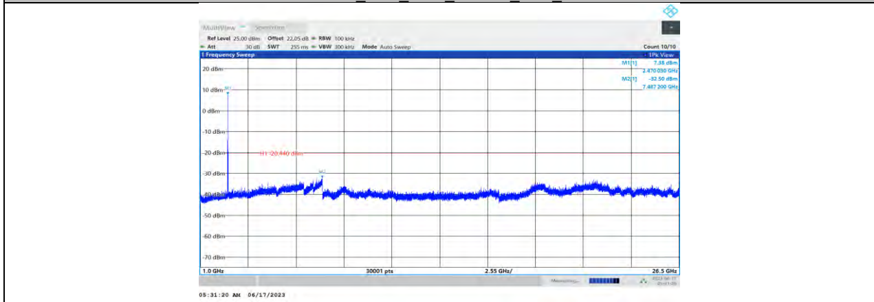
11AX20MIMO_Ant0_2462_26Tone_RU8_1000~26500
