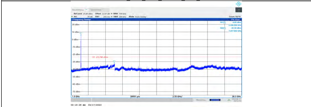
11AX40MIMO_Ant0_2437_26Tone_RU8_1000~26500
