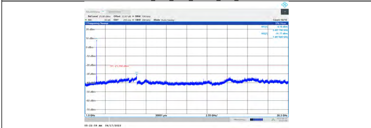
11AX20MIMO_Ant0_2437_26Tone_RU4_1000~26500
