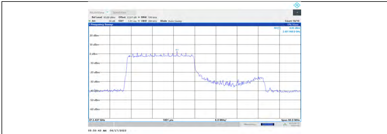
11AX40MIMO_Ant0_2437_242Tone_RU61_0~Reference
