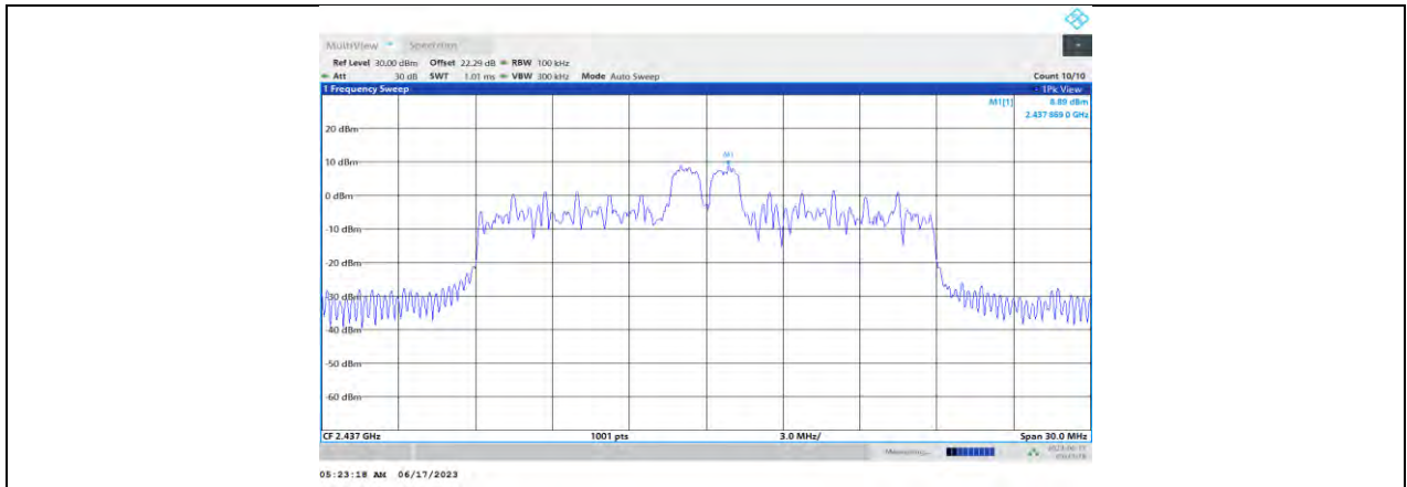
11AX20MIMO_Ant1_2437_26Tone_RU4_0~Reference
