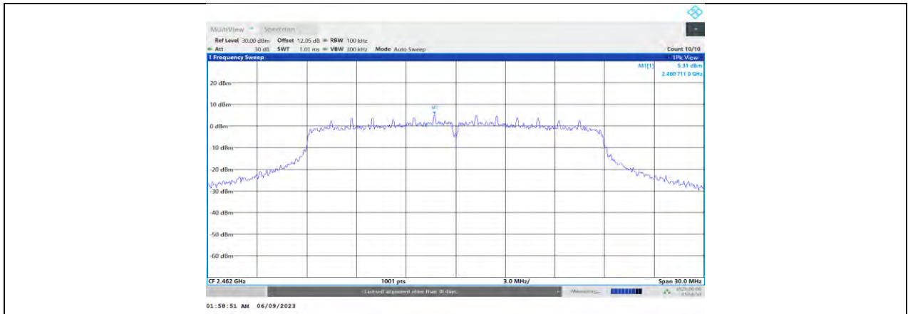
11N20MIMO_Ant0_2462_0~Reference
