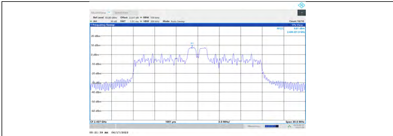
11AX20MIMO_Ant0_2437_26Tone_RU4_0~Reference
