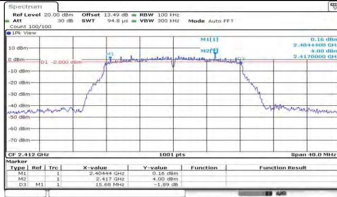
11G Ant1 2412
