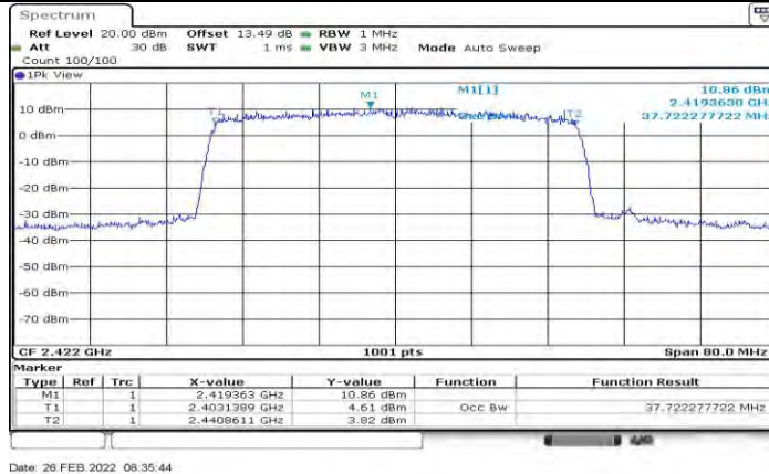
11AX40MIMO Ant2_2422
