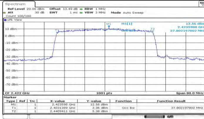
11AX40MIMO Ant1_2422
