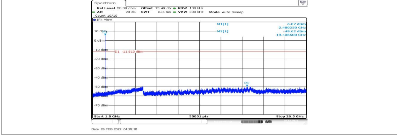
BLE_2M_Ant1_2480_1000~26500
