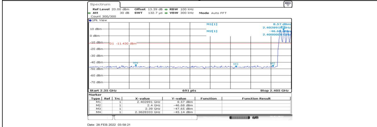
DH5_Ant1_Low_Hop_2402
