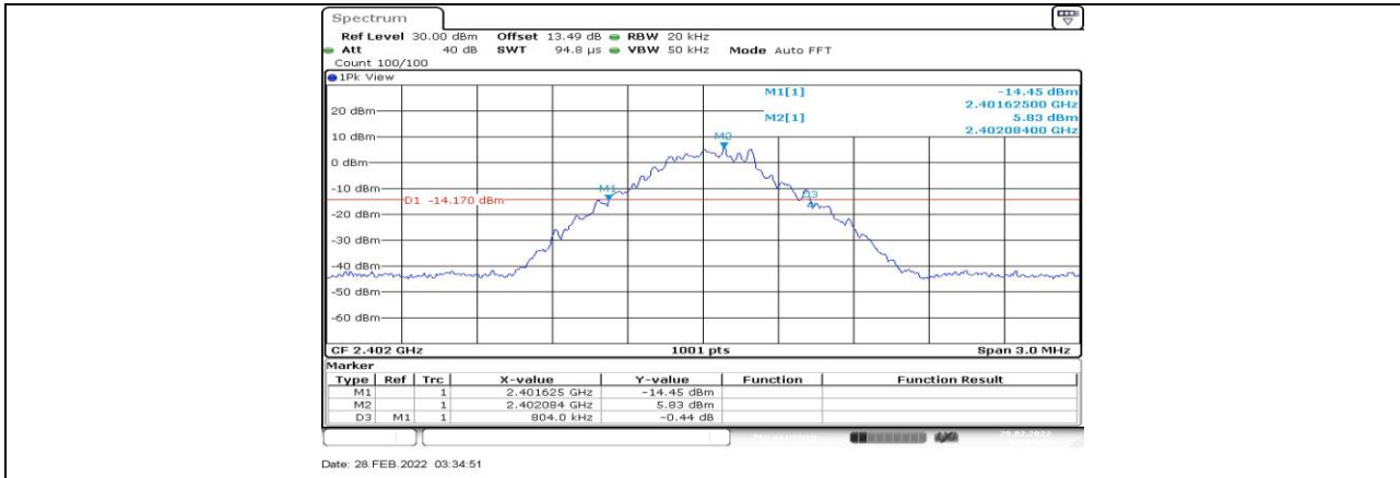
DH5_Ant1_2402
