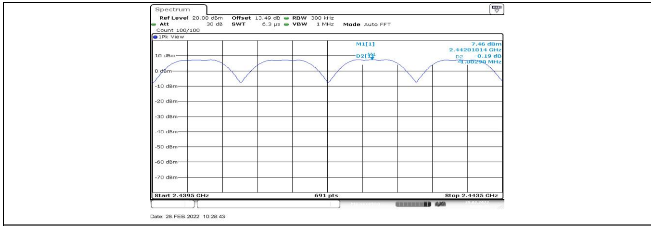
DH5_Ant1_Hop
