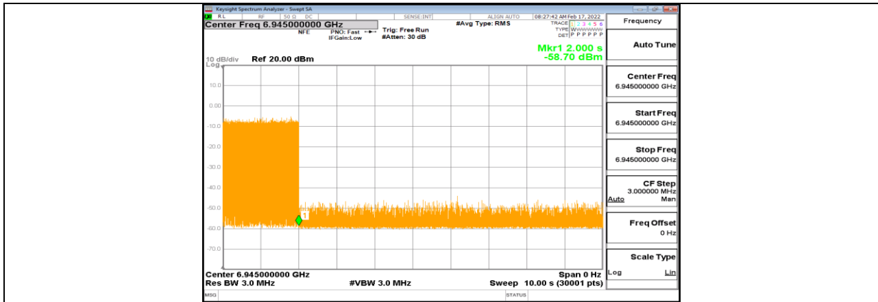
11AX80MIMO_Ant1_6945_Center_6945_4
