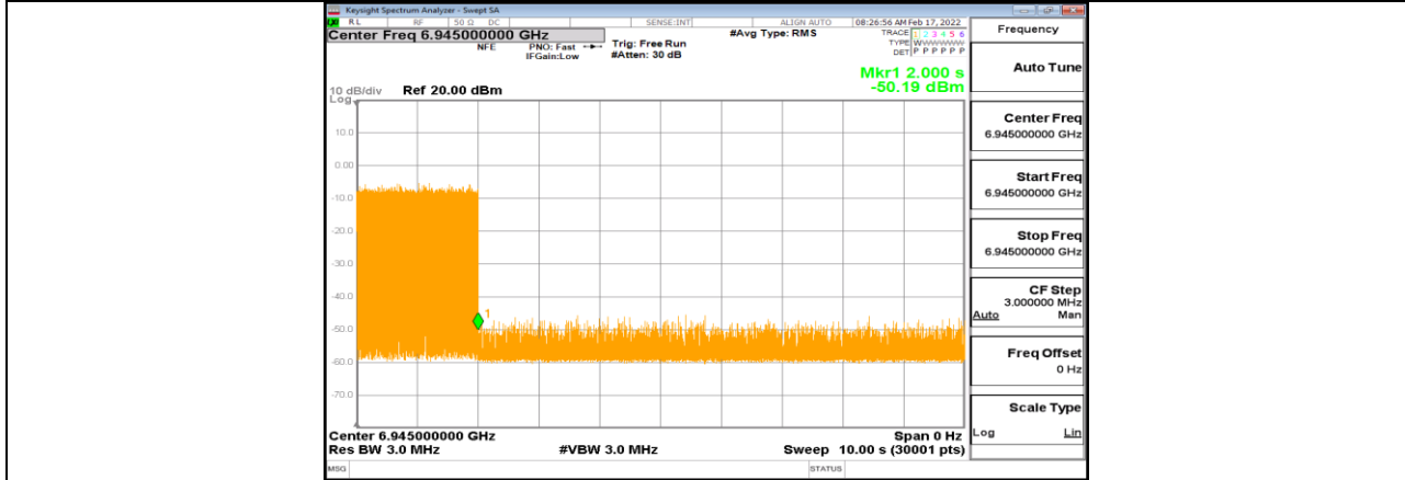
11AX80MIMO_Ant1_6945_Center_6945_3
