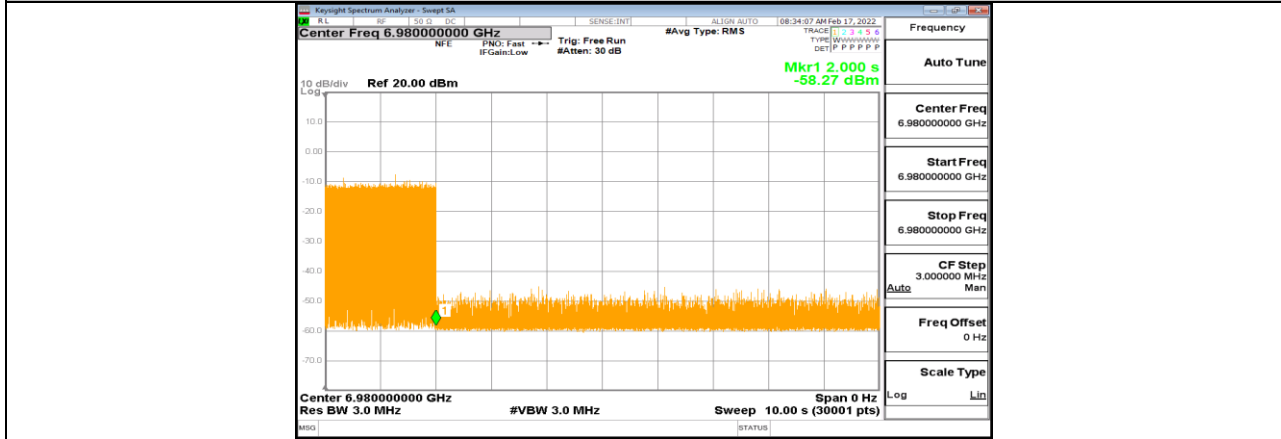
11AX80MIMO_Ant1_6945_Low_6980_1
