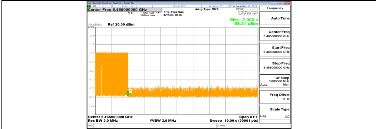
11AX80MIMO_Ant1_6465_Center_6465_5
