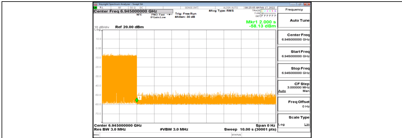
11AX80MIMO_Ant1_6945_Center_6945_1
