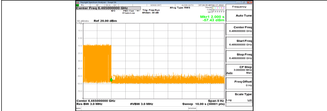
11AX80MIMO_Ant1_6465_Center_6465_9
