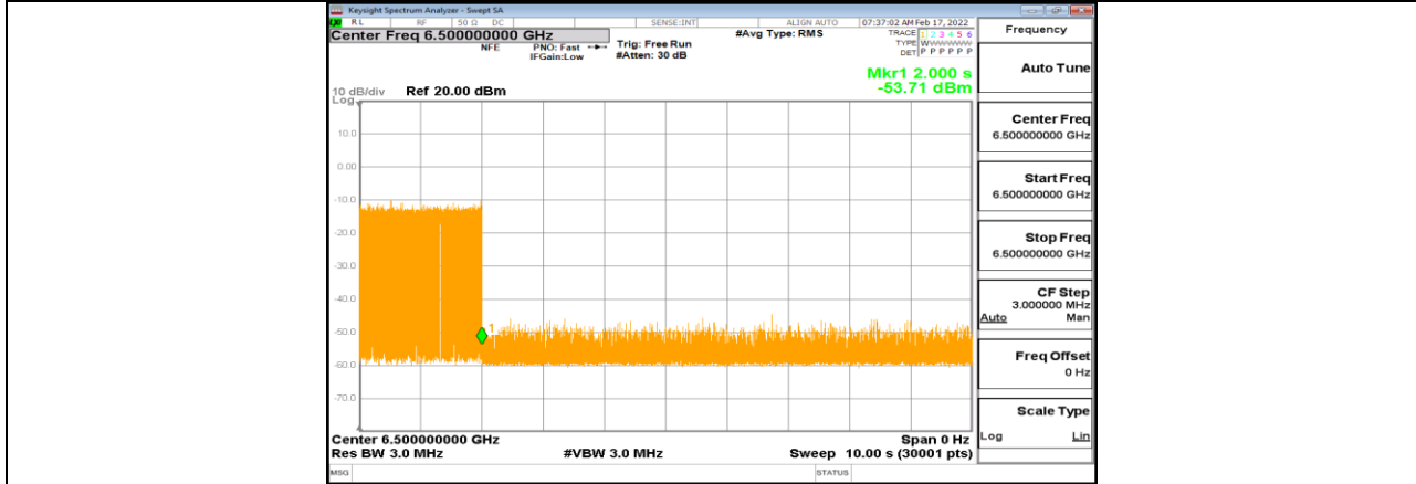
11AX80MIMO_Ant1_6465_Low_6500_2
