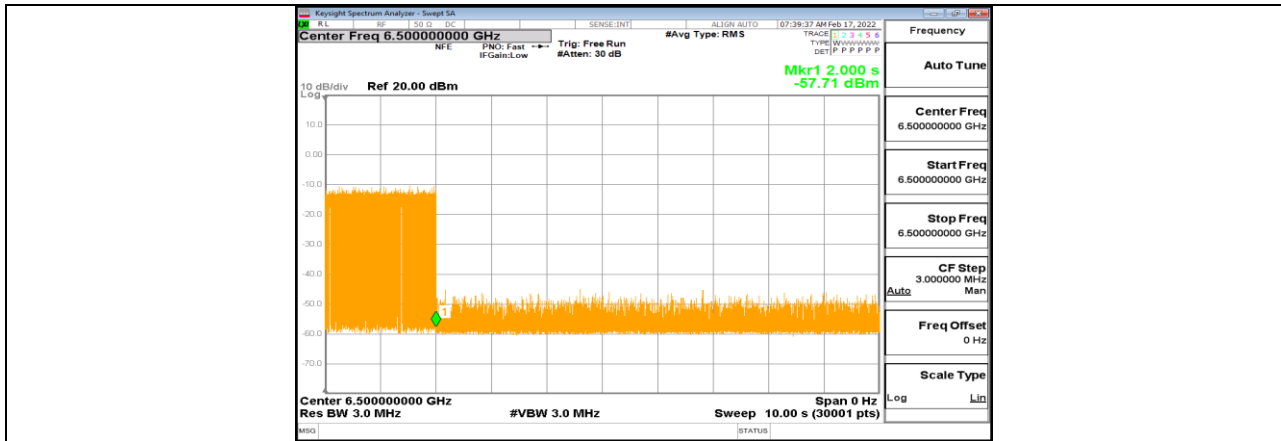
11AX80MIMO_Ant1_6465_Low_6500_6
