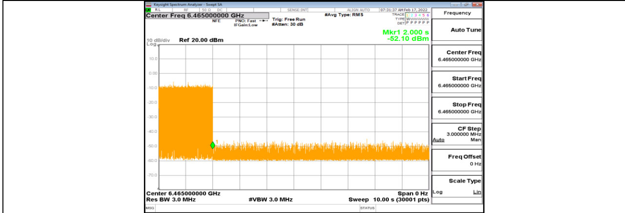
11AX80MIMO_Ant1_6465_Center_6465_6
