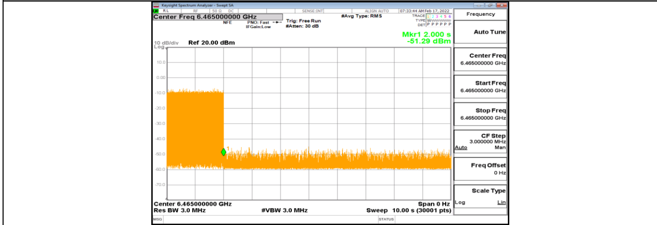
11AX80MIMO_Ant1_6465_Center_6465_8
