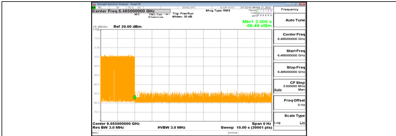
11AX80MIMO_Ant1_6465_Center_6465_7
