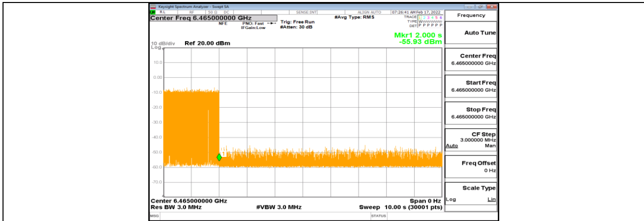
11AX80MIMO_Ant1_6465_Center_6465_1
