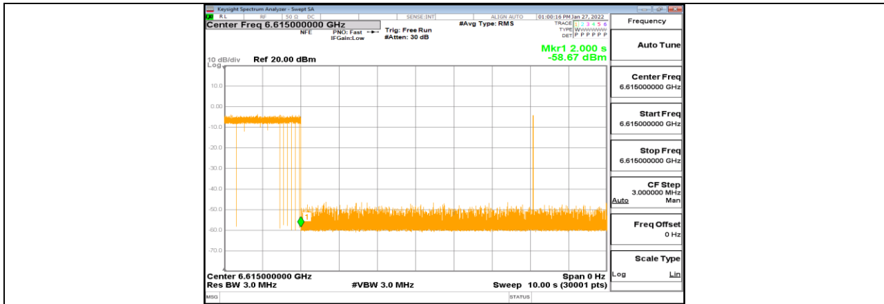
11AX20MIMO_Ant1_6615_Center_6615_7
