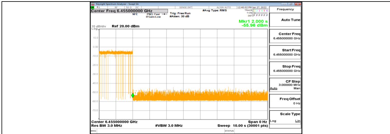
11AX20MIMO_Ant1_6455_Center_6455_2
