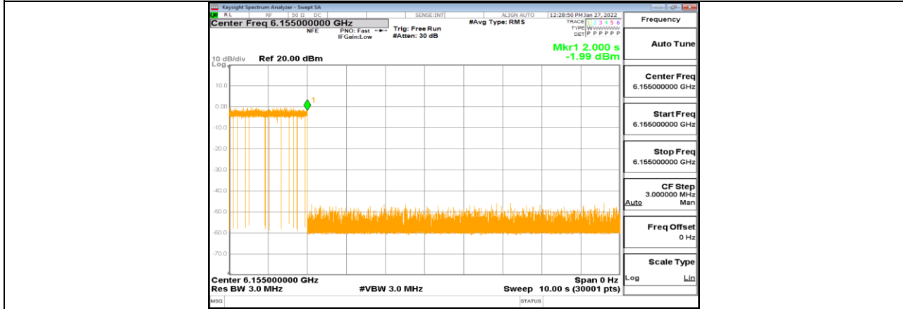
11AX20MIMO_Ant1_6155_Center_6155_4
