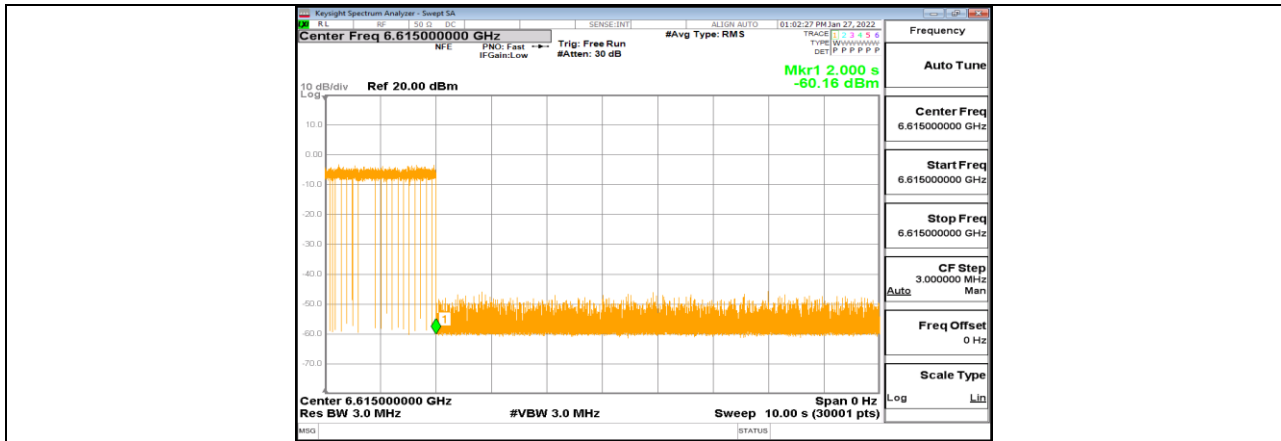
11AX20MIMO_Ant1_6615_Center_6615_10
