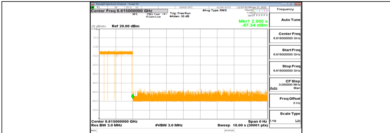
11AX20MIMO_Ant1_6615_Center_6615_1
