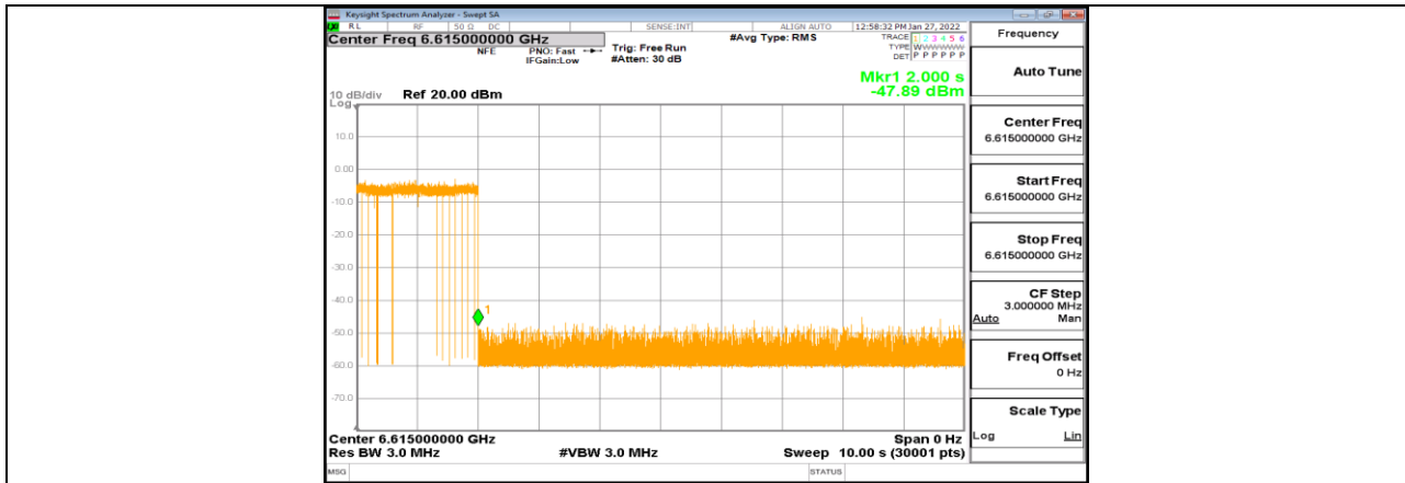
11AX20MIMO_Ant1_6615_Center_6615_4
