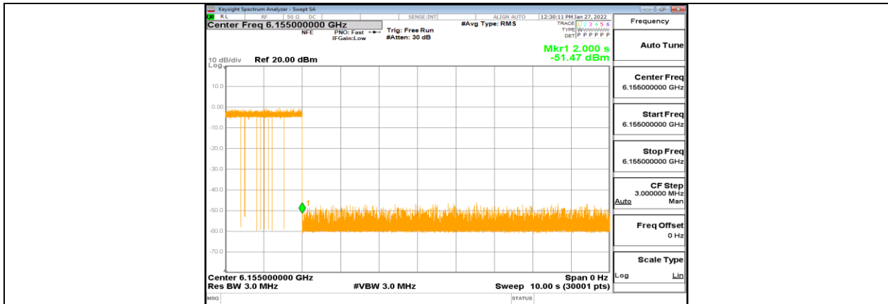
11AX20MIMO_Ant1_6155_Center_6155_6
