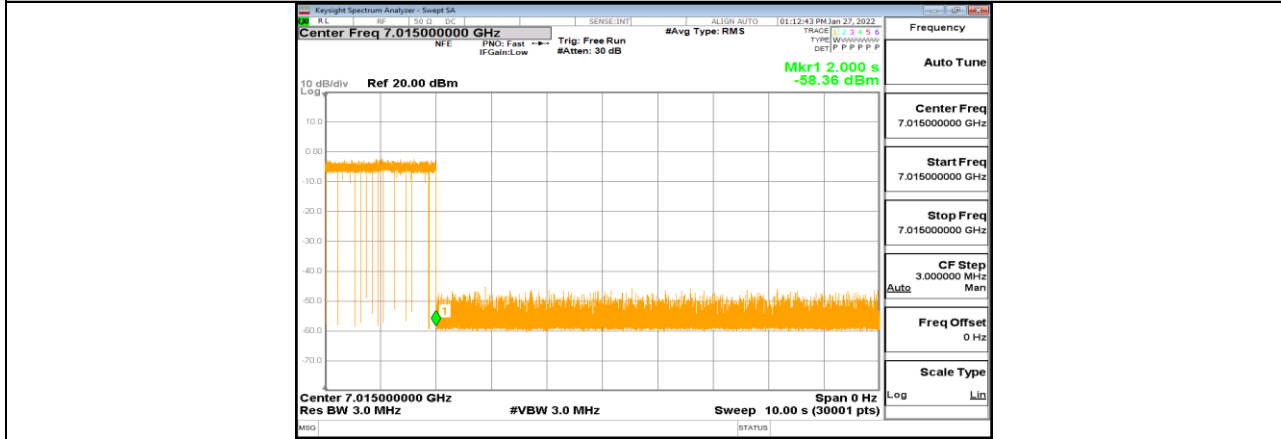
11AX20MIMO_Ant1_7015_Center_7015_4
