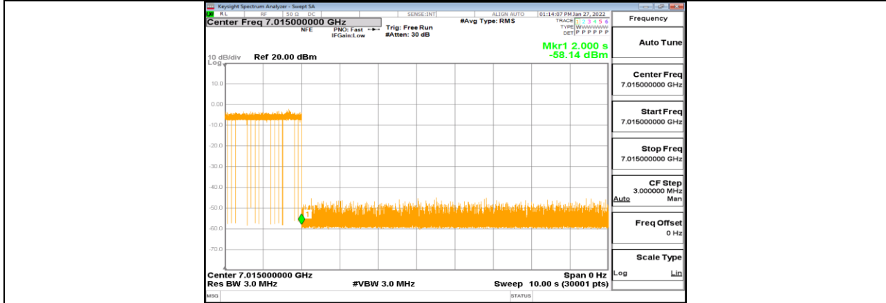
11AX20MIMO_Ant1_7015_Center_7015_5
