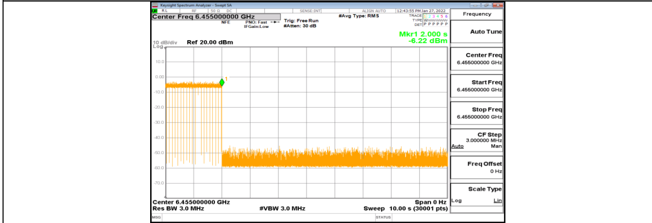
11AX20MIMO_Ant1_6455_Center_6455_9
