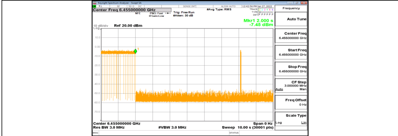
11AX20MIMO_Ant1_6455_Center_6455_7
