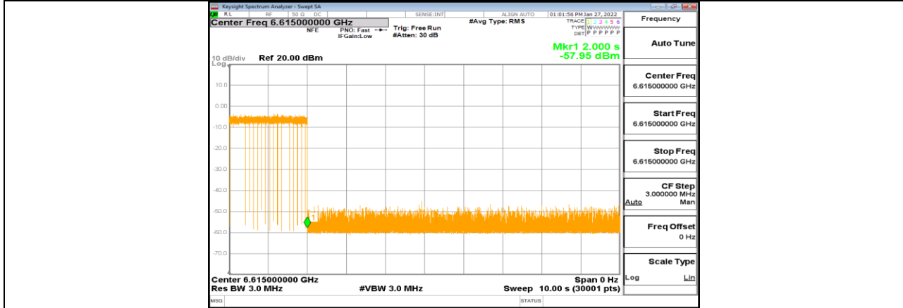
11AX20MIMO_Ant1_6615_Center_6615_9
