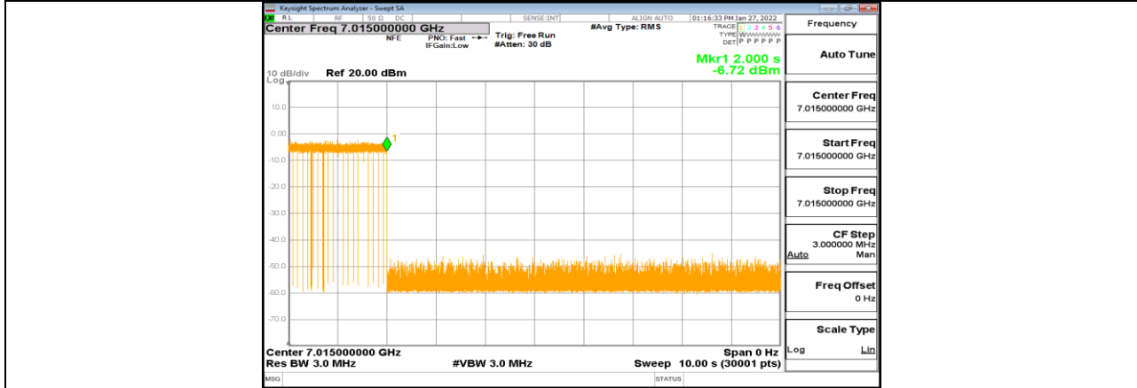
11AX20MIMO_Ant1_7015_Center_7015_8
