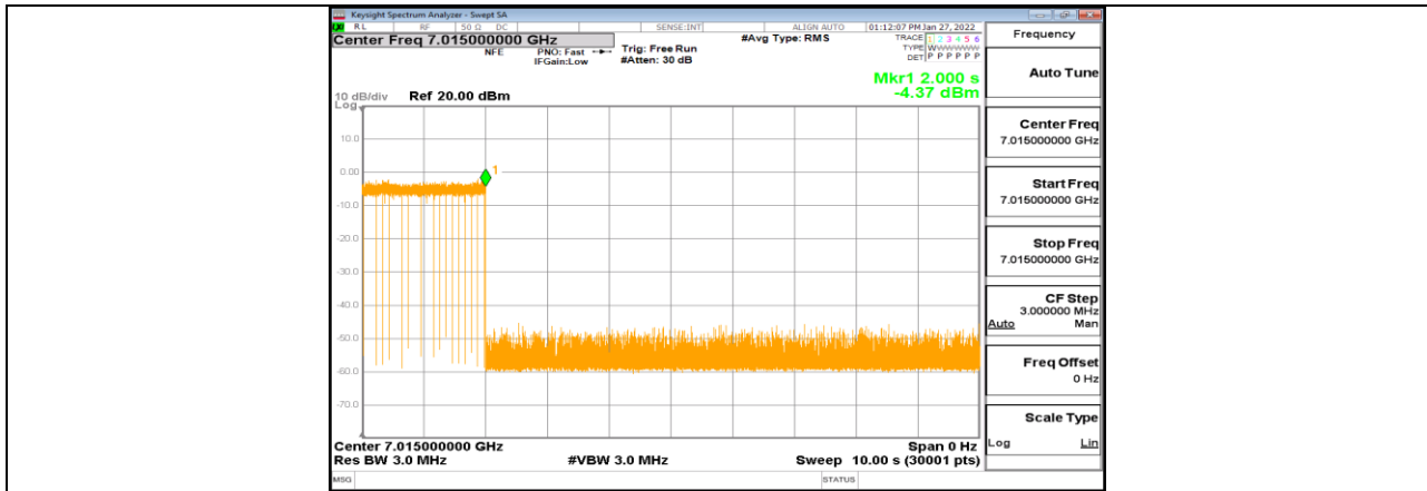
11AX20MIMO_Ant1_7015_Center_7015_3
