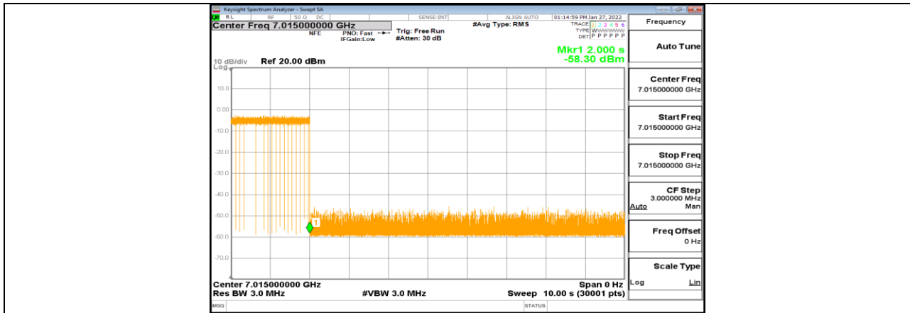
11AX20MIMO_Ant1_7015_Center_7015_6
