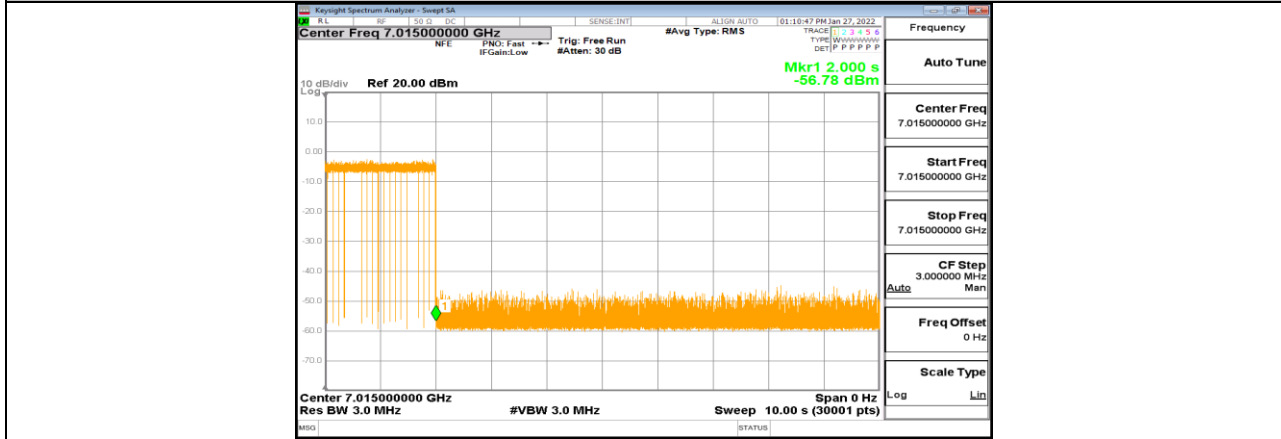
11AX20MIMO_Ant1_7015_Center_7015_1
