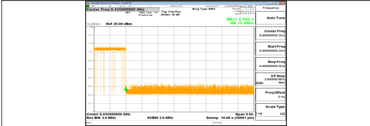
11AX20MIMO_Ant1_6455_Center_6455_6
