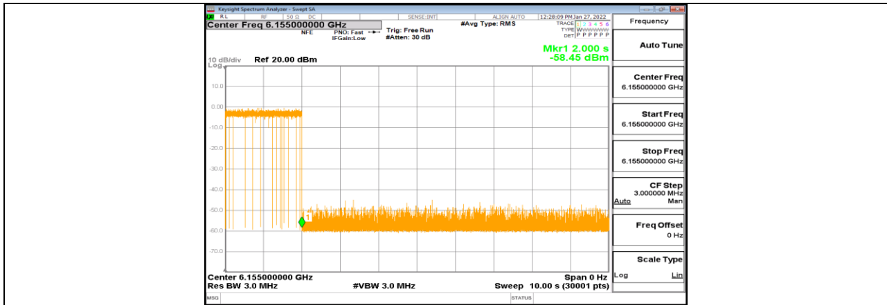
11AX20MIMO_Ant1_6155_Center_6155_3
