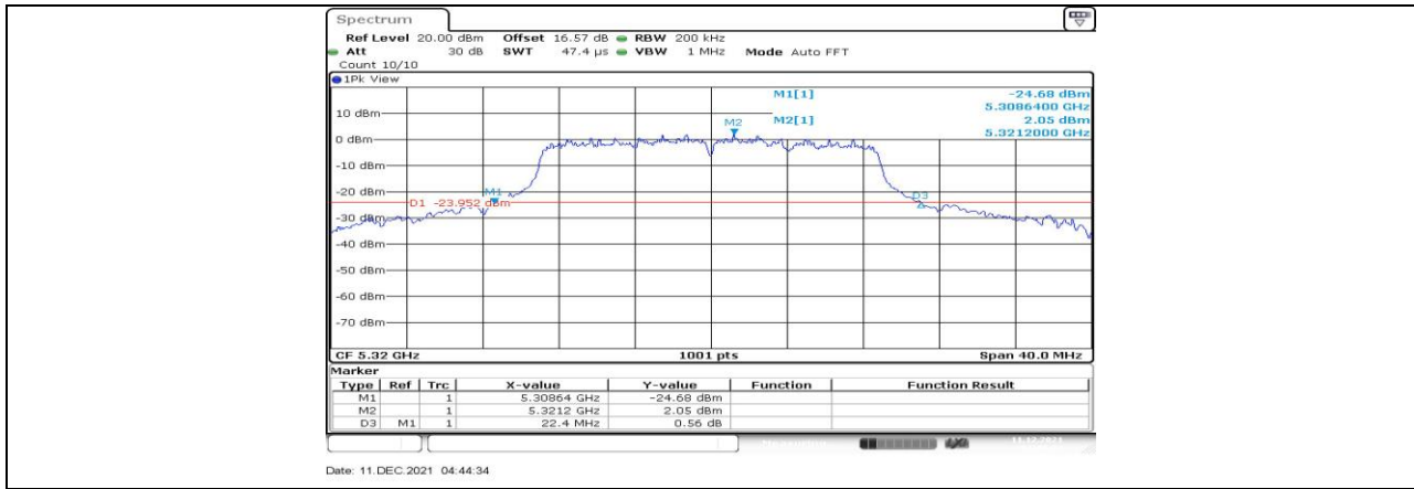
11AC20MIMO_Ant1_5320
