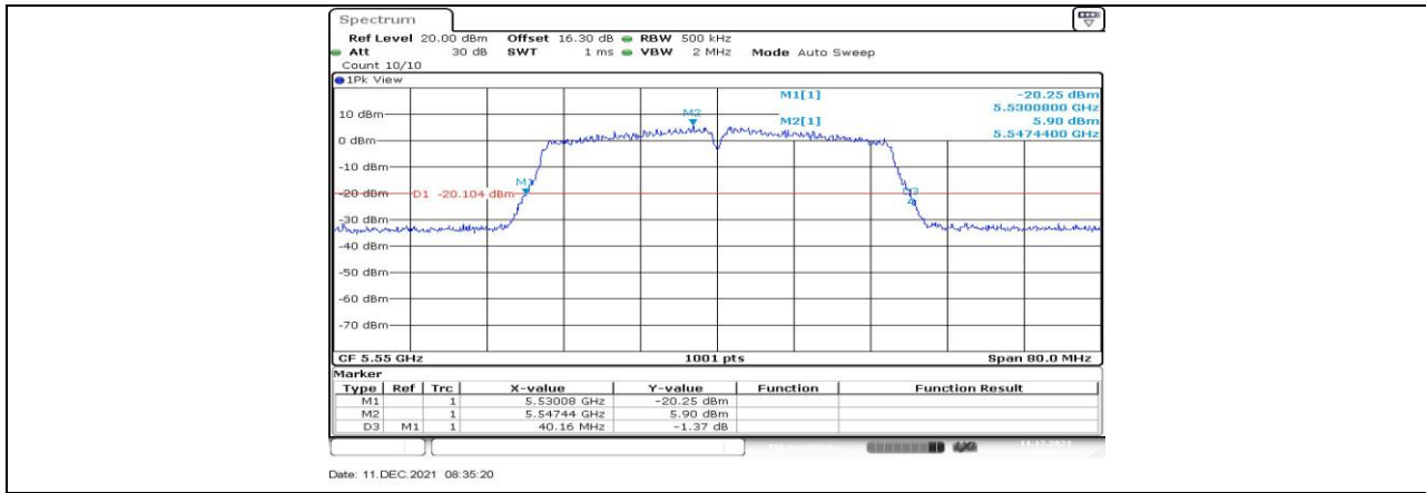
11AC40MIMO_Ant2_5550
