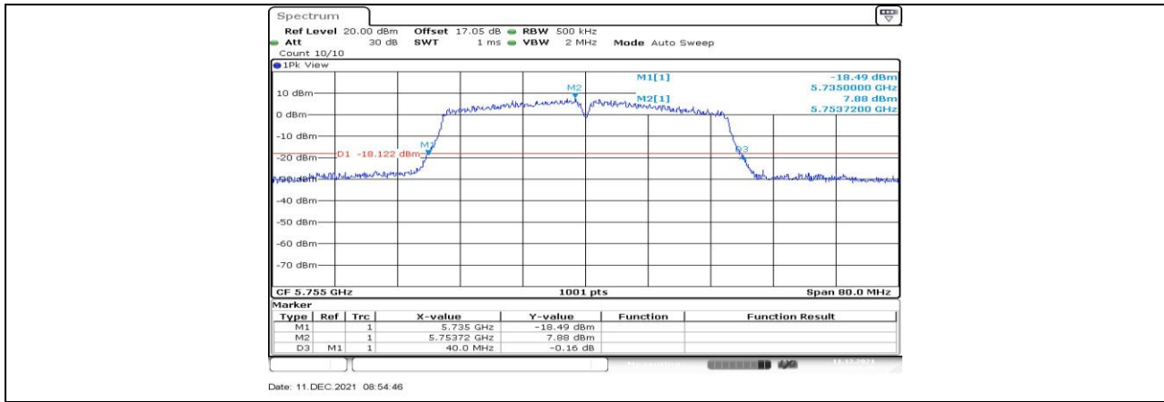
11AC40MIMO_Ant2_5755
