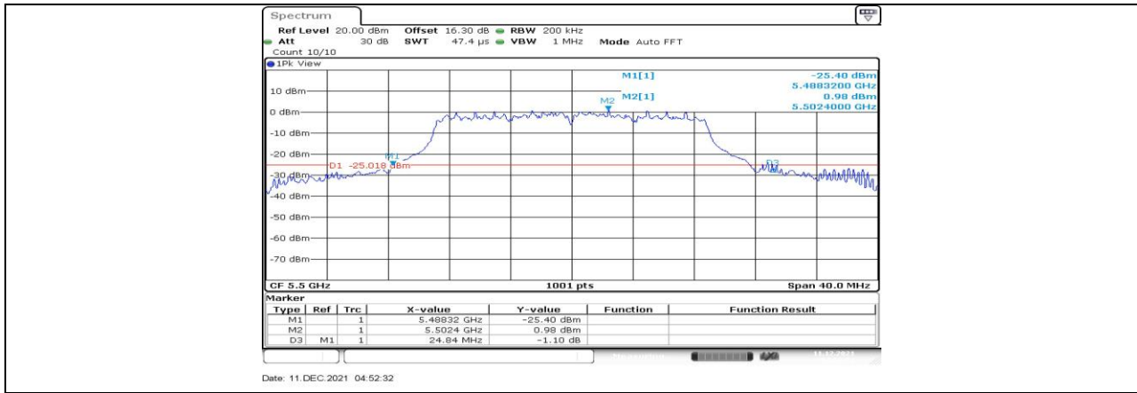
11AC20MIMO_Ant2_5500
