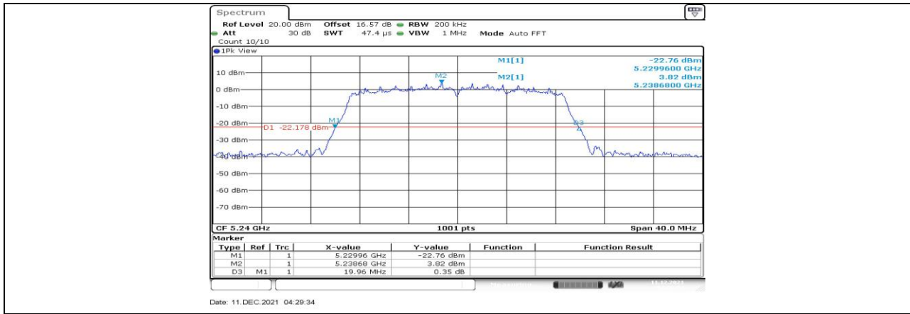
11AC20MIMO_Ant1_5240
