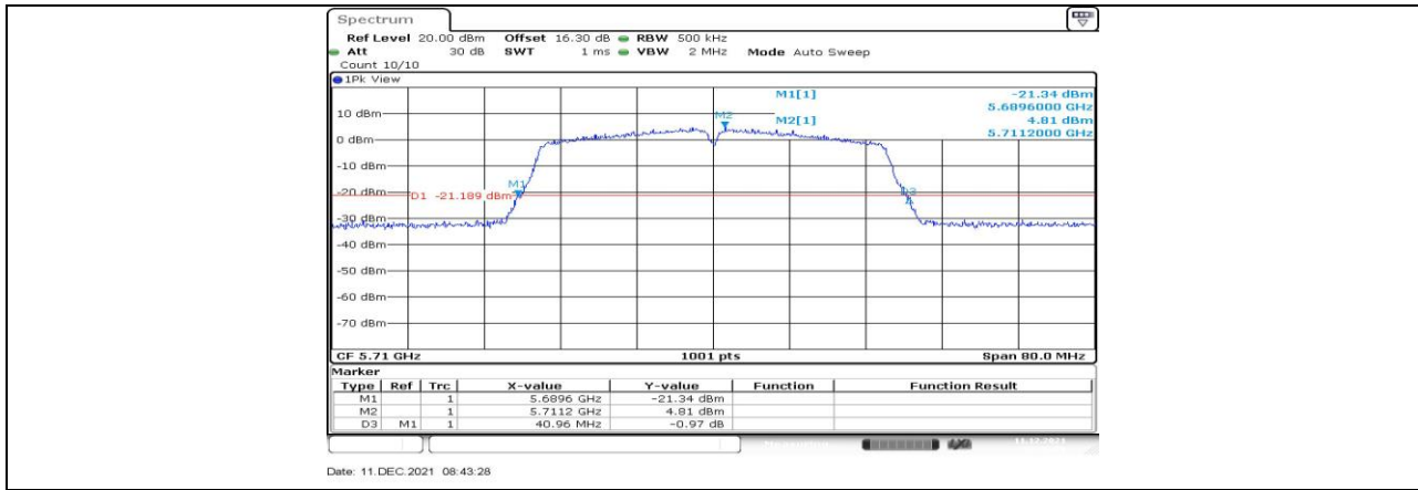
11AC40MIMO_Ant1_5710
