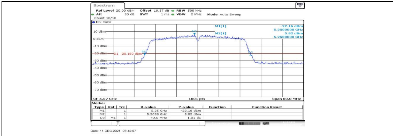
11AC40MIMO_Ant2_5270
