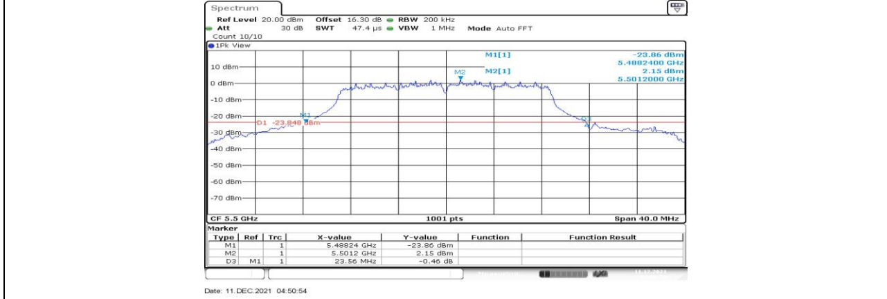
11AC20MIMO_Ant1_5500
